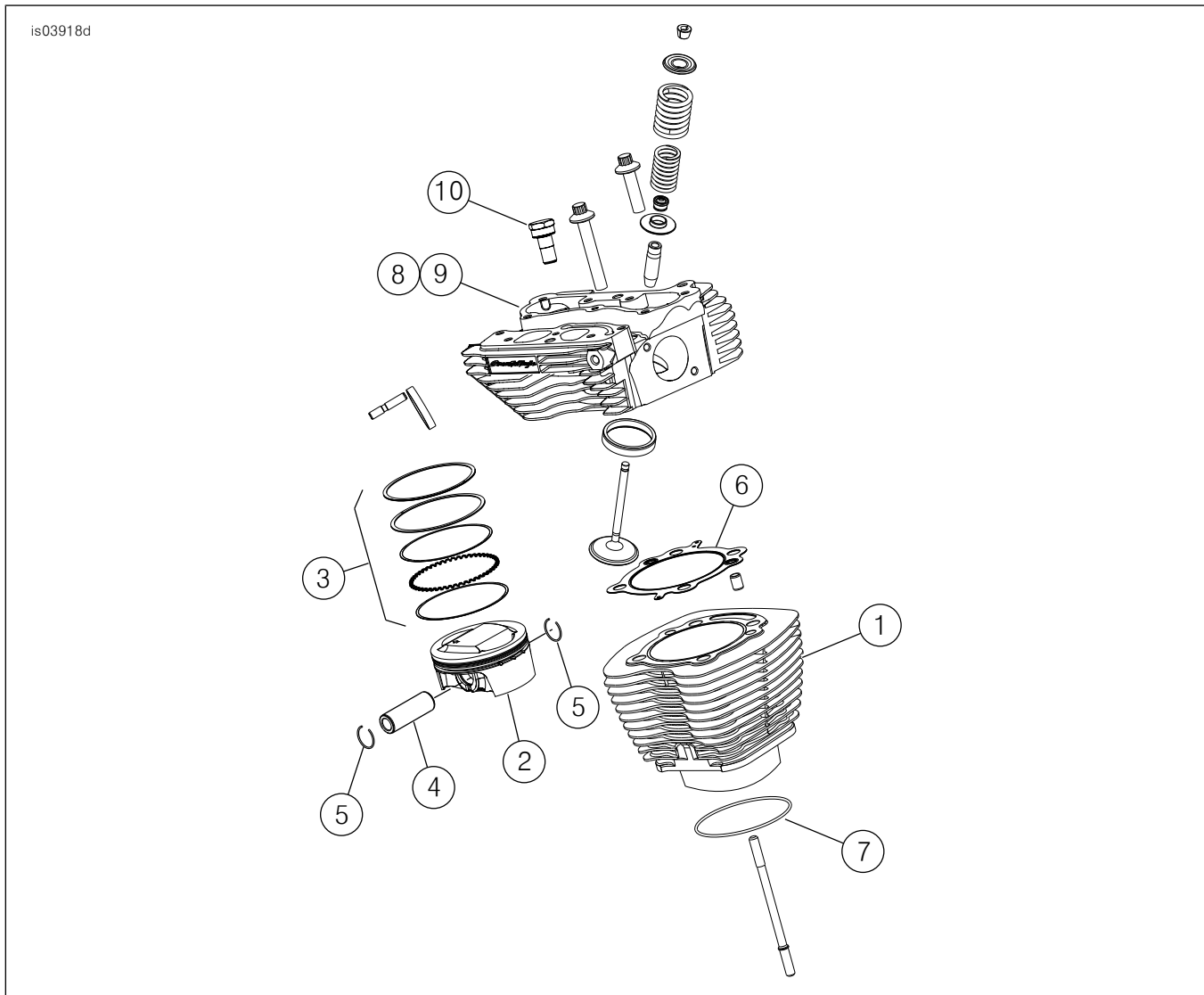
그림 1. 정비 부품: Screamin' Eagle Pro TC 103(96 CI ~ 103 CI) 스테이지 4 키트
