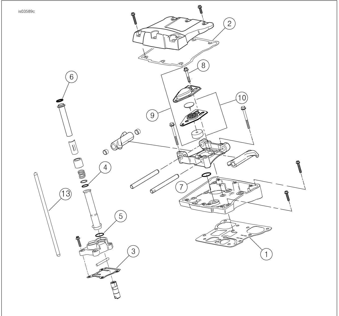
그림 2. 정비 부품: Screamin' Eagle Pro TC 103(96 CI ~ 103 CI) 스테이지 4 키트
