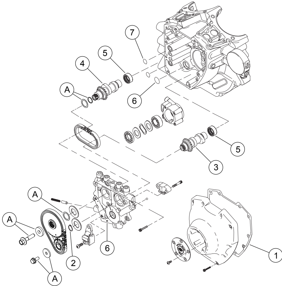
그림 3. 정비 부품: Screamin' Eagle Pro TC 103(96 CI ~ 103 CI) 스테이지 4 키트
