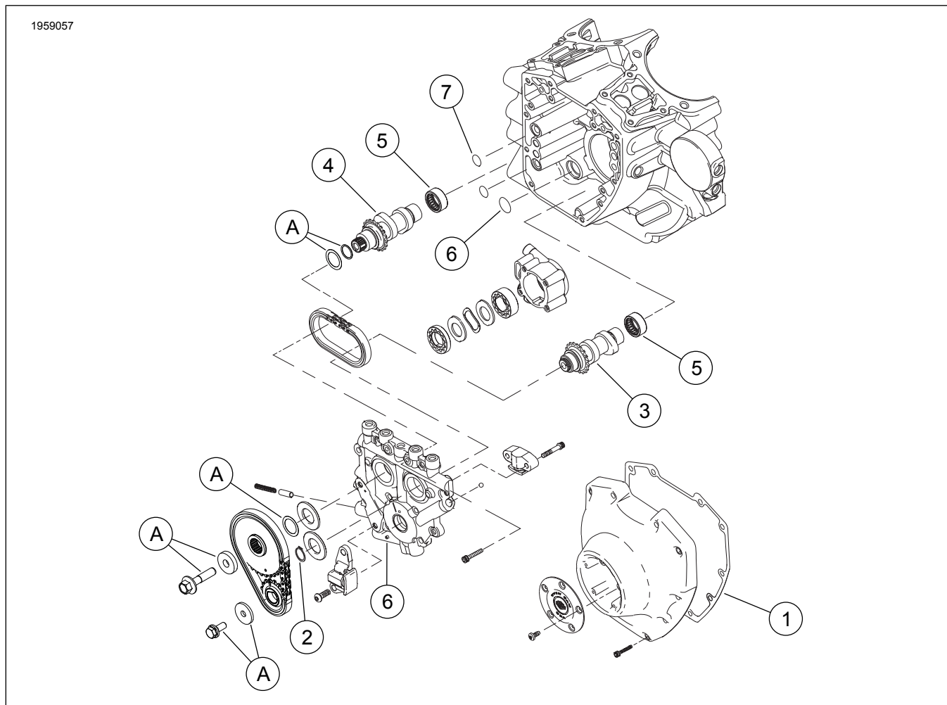
Slika 3. Servisni deli: Komplet Screamin' Eagle Pro TC 103 (96 CI do 103 CI) Stage 4
