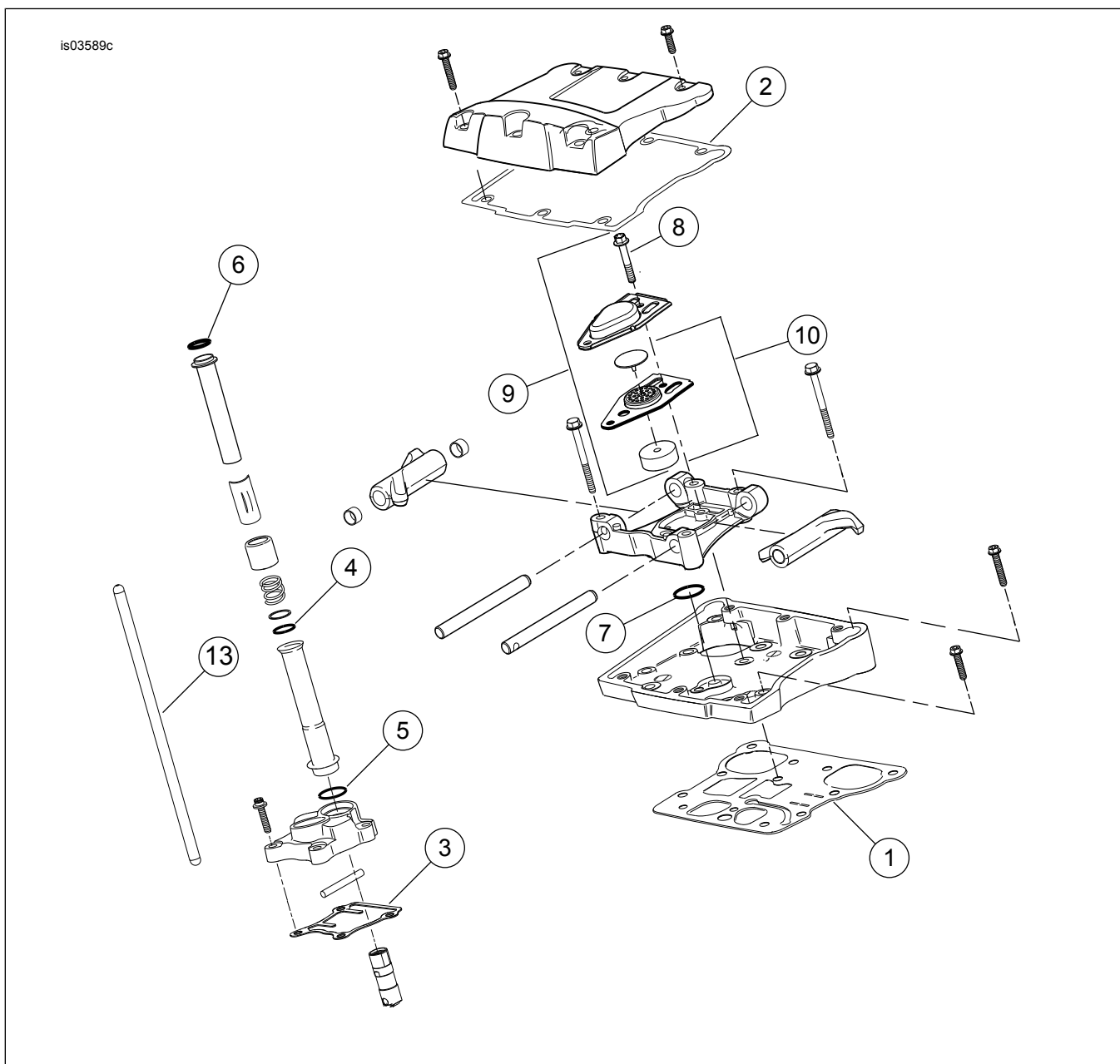
Pav 2. Dalys, reikalingos užduočiai atlikti "Screamin' Eagle Pro" TC 103 (nuo 96 iki 103 CI) 4 etapo komplektas
