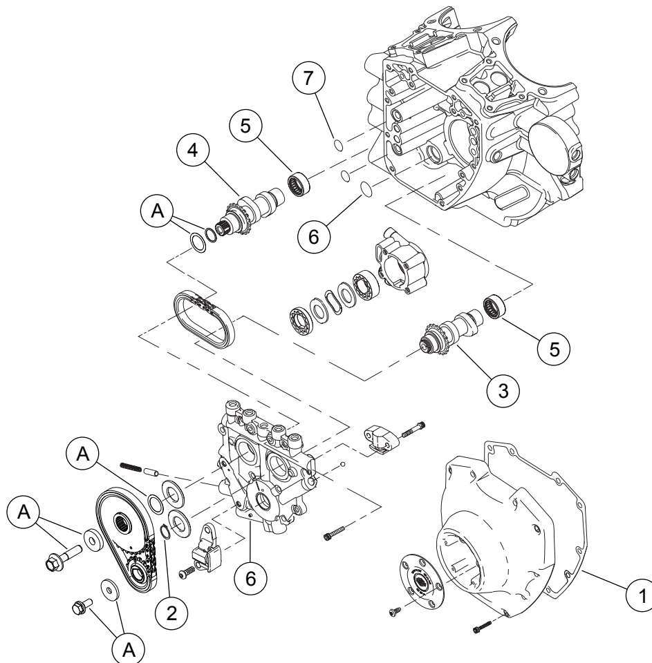
Pav 3. Dalys, reikalingos užduočiai atlikti "Screamin' Eagle Pro" TC 103 (nuo 96 iki 103 CI) 4 etapo komplektas
