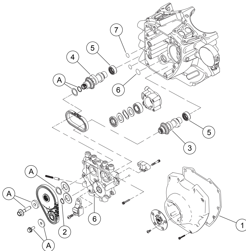
Εικόνα 3. Ανταλλακτικά: Κιτ Screamin' Eagle Pro TC 103 (96 CI έως 103 CI) Στάδιο 4
