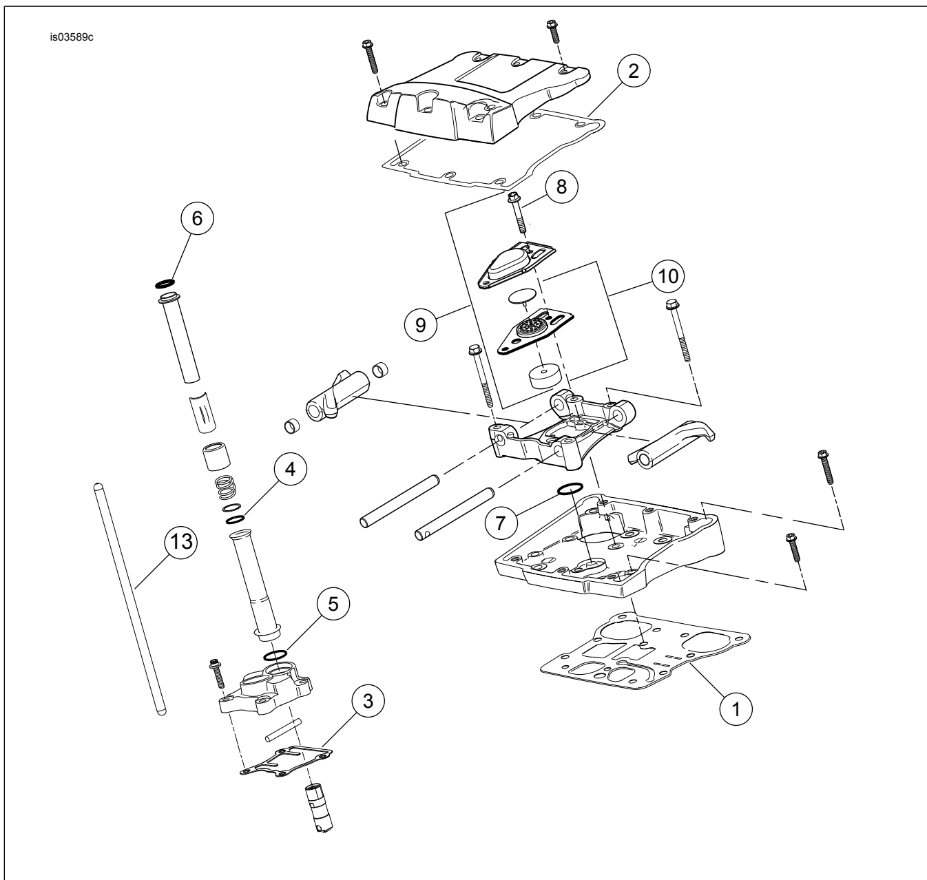
Εικόνα 2. Ανταλλακτικά: Κιτ Screamin' Eagle Pro TC 103 (96 CI έως 103 CI) Στάδιο 4
