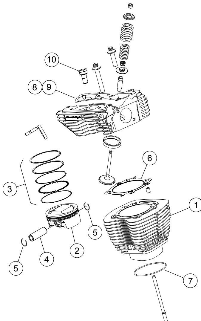
Slika 1. Servisni dijelovi: Screamin' Eagle Pro TC 103 (96 CI do 103 CI) Stage 4 komplet
