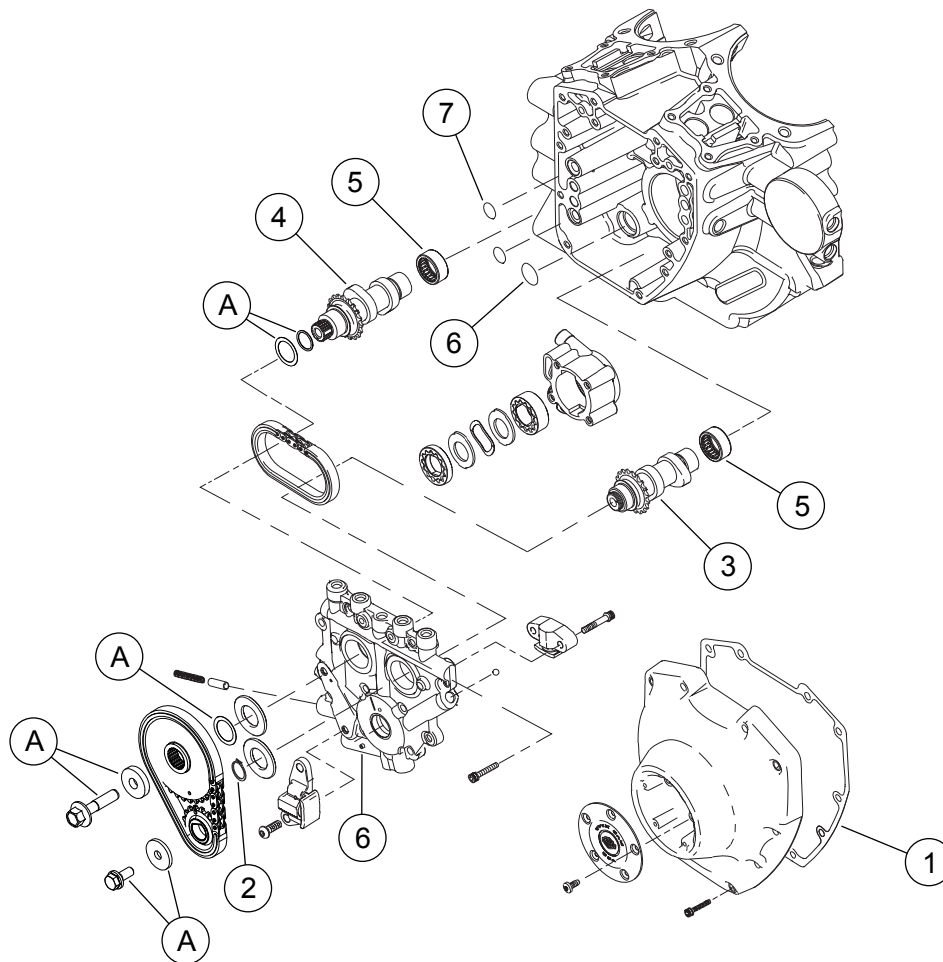
Slika 3. Servisni dijelovi: Screamin' Eagle Pro TC 103 (96 CI do 103 CI) Stage 4 komplet
