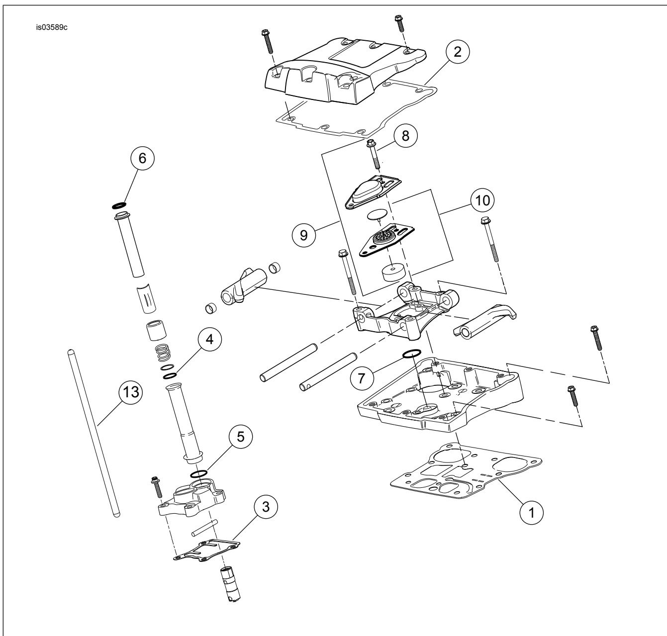
Slika 2. Servisni dijelovi: Screamin' Eagle Pro TC 103 (96 CI do 103 CI) Stage 4 komplet
