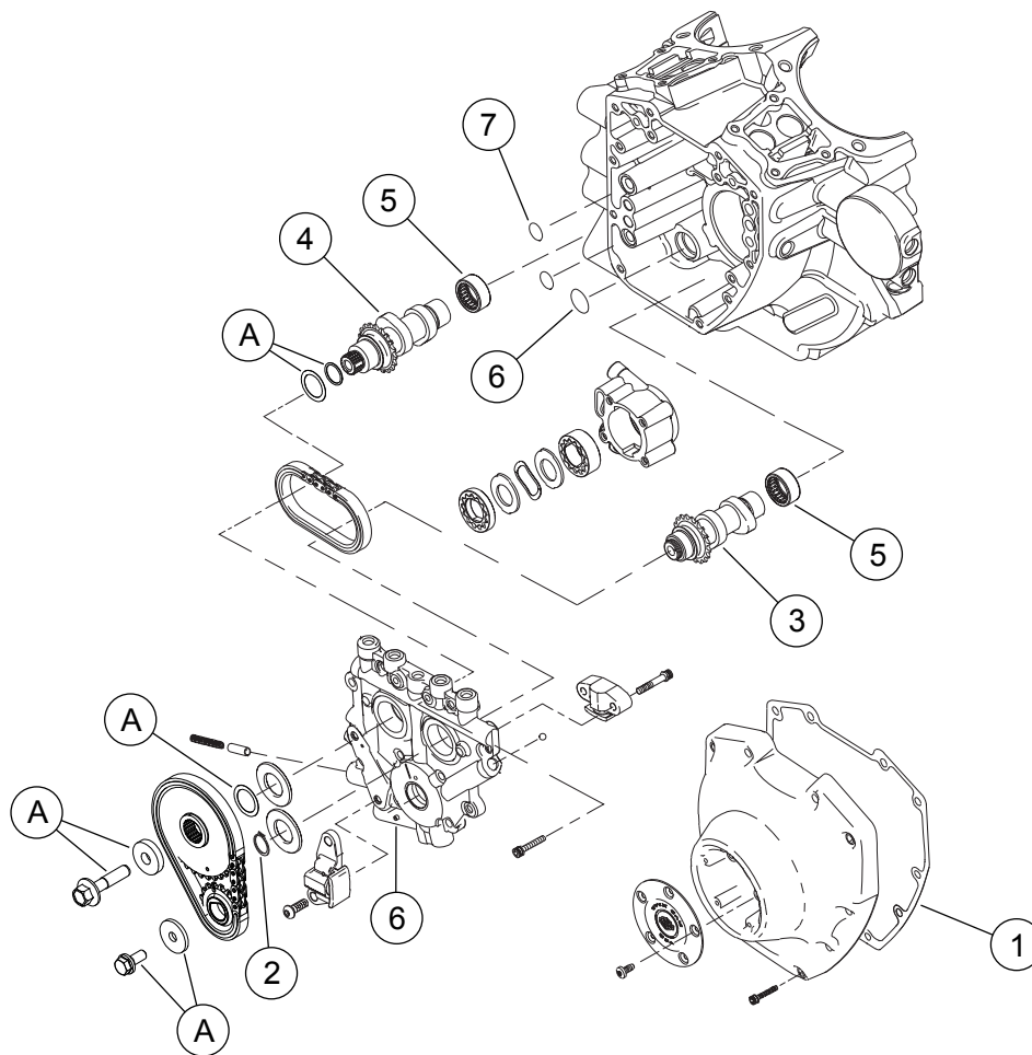
Figur 3. Servicedeler: Screamin' Eagle Pro TC 103 (96 CI til 103 CI) Stage 4-sett
