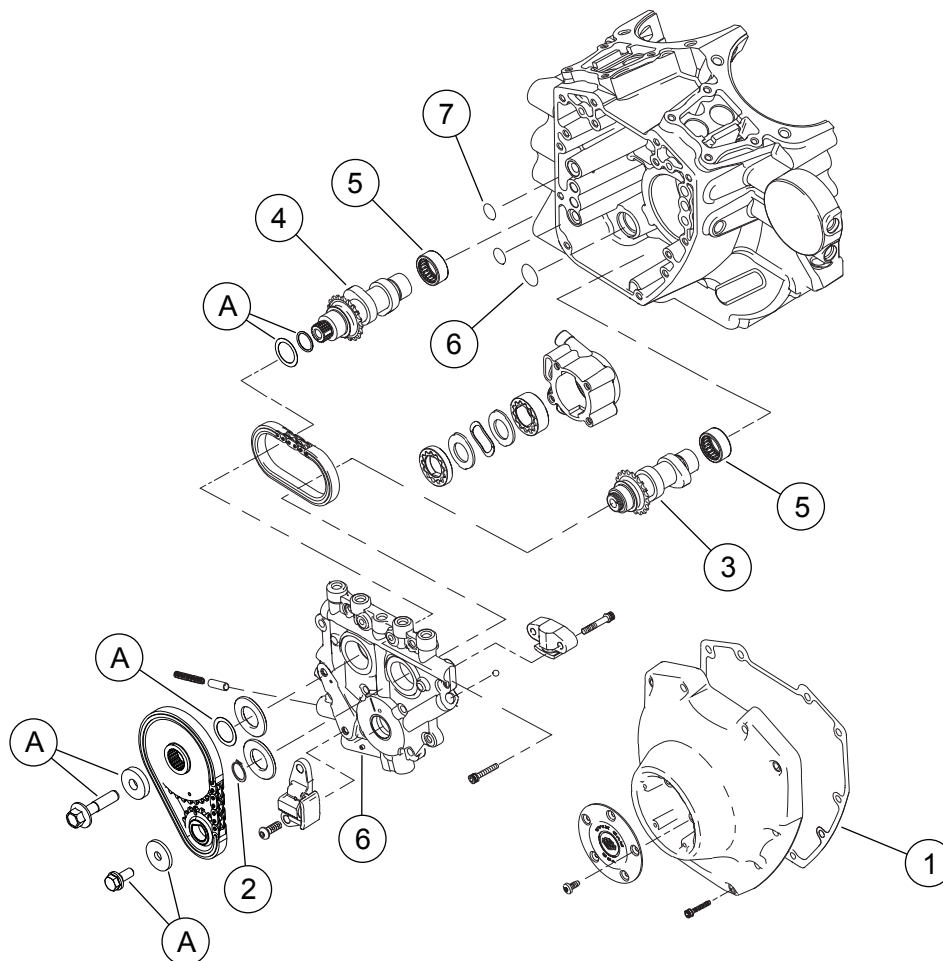
Figur 3. Reservedele: Screamin' Eagle Pro TC 103 (96 CI til 103 CI) Trin 4 sæt
