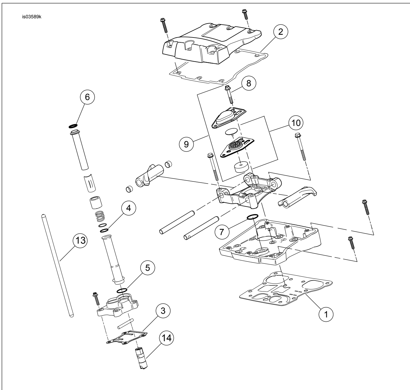
Figure 2. Mga Pamalit na Piyesa: Screamin' Eagle Pro TC 103 CI Stage 4 Kit
