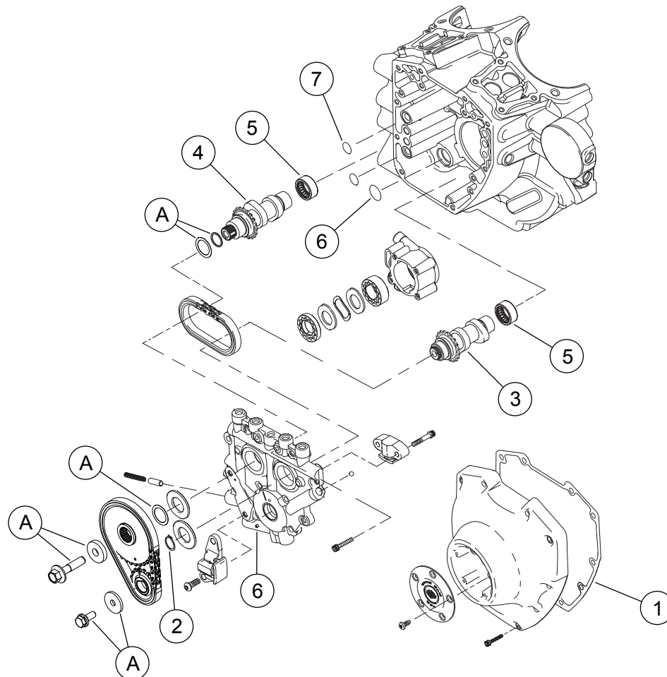
תרשים 3. חלקי שירות: ערכת Screamin' Eagle Pro TC 103 CI שלב 4
