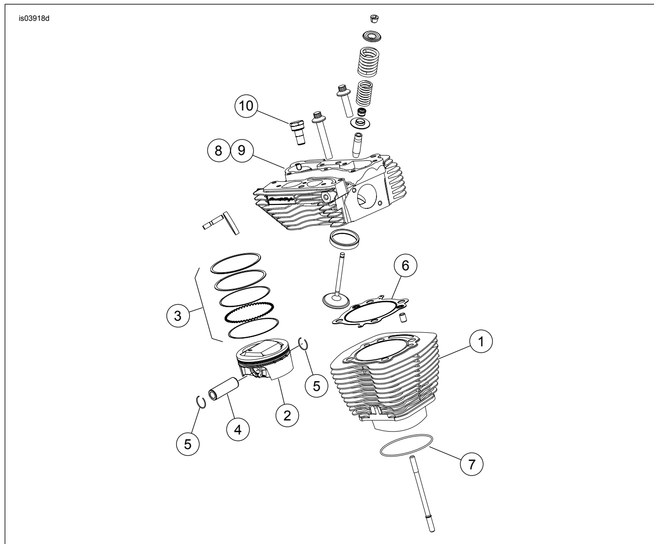
תרשים 1. חלקי שירות: ערכת Screamin' Eagle Pro TC 103 Cl שלב 4
