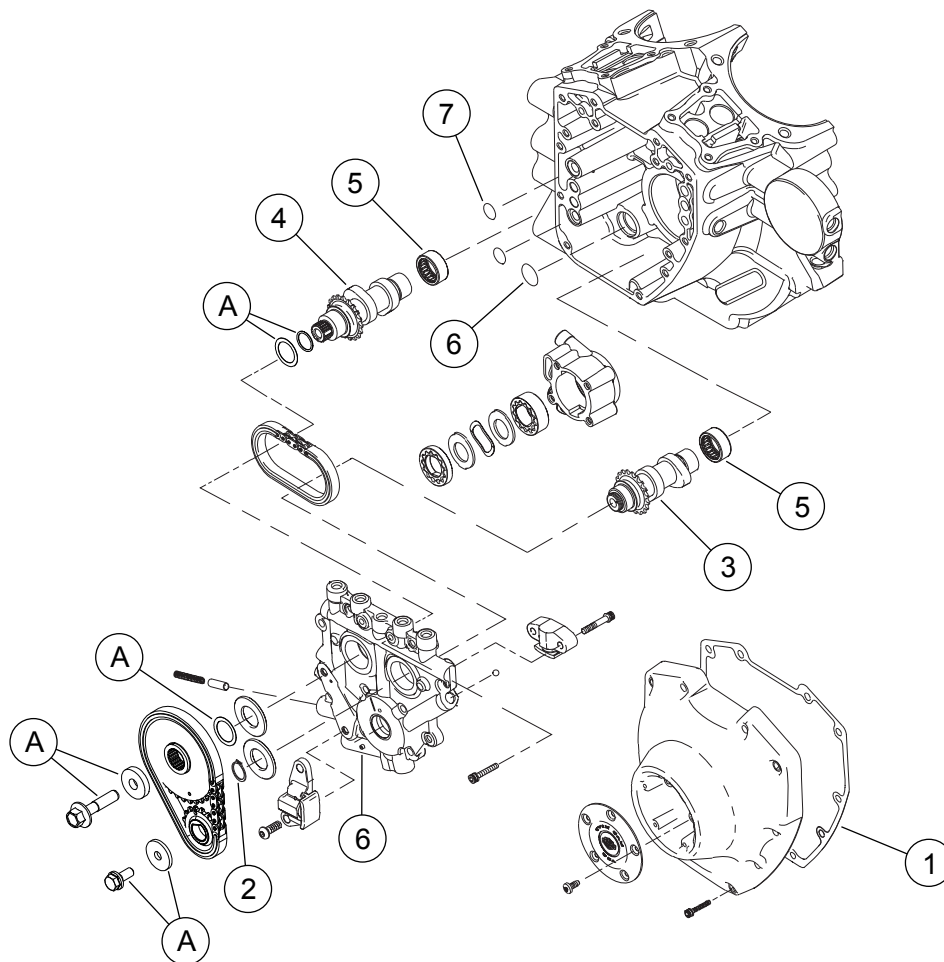
Ilustrace 3. Servisní díly: Sada Screamin' Eagle Pro TC 103 in3 Stage 4
