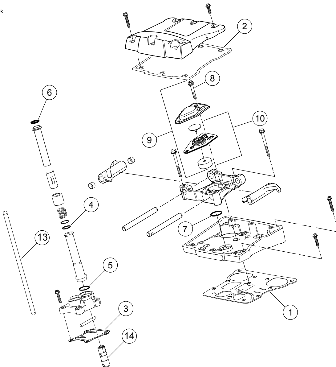
Ilustrace 2. Servisní díly: Sada Screamin' Eagle Pro TC 103 in3 Stage 4
