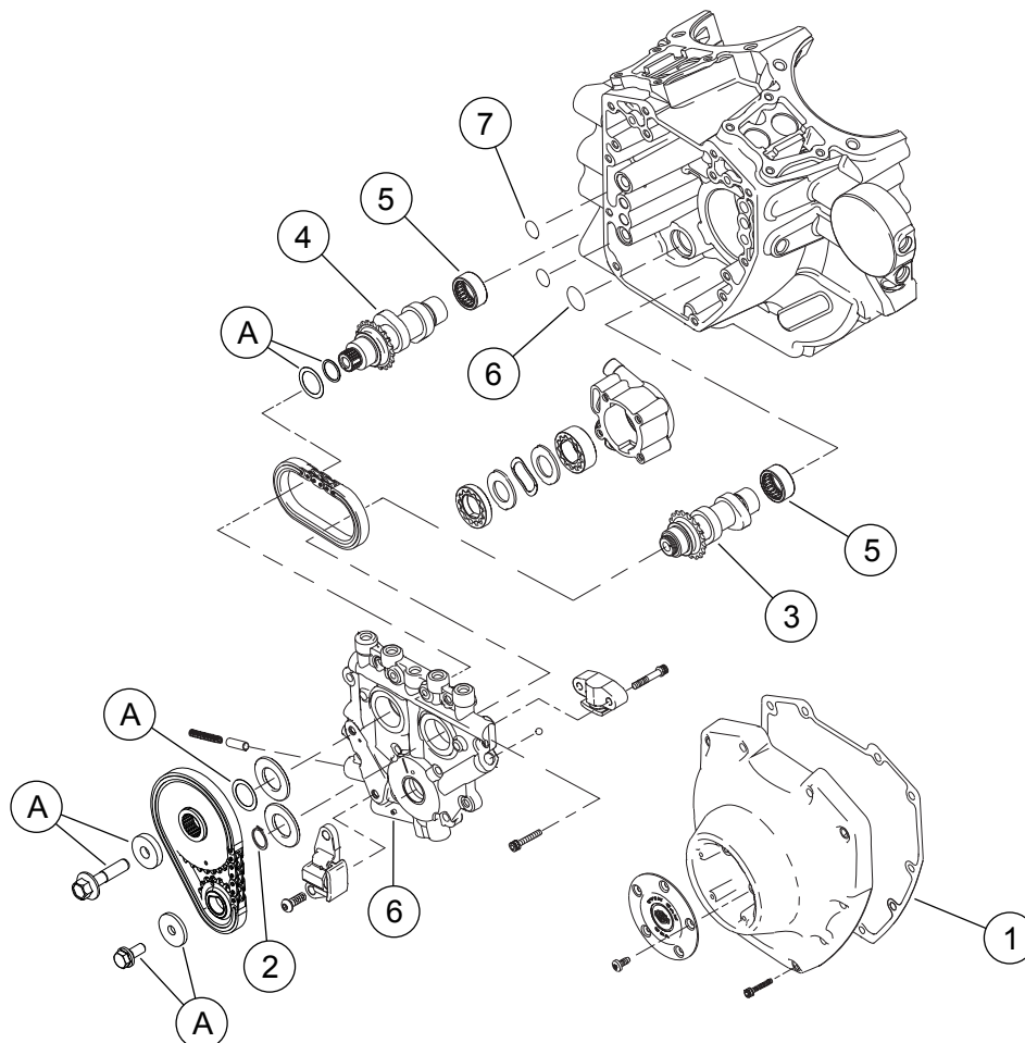
Pav 3. Dalys, reikalingos užduočiai atlikti "Screamin' Eagle Pro" TC 103 CI 4 etapo komplektas
