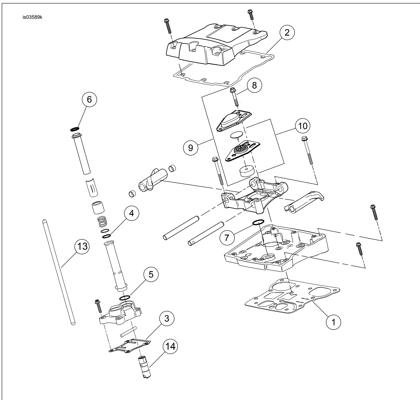
Рисунок 2. Запасные части: Комплект 4 ступени для двигателя Screamin' Eagle Pro TC 103 CI
