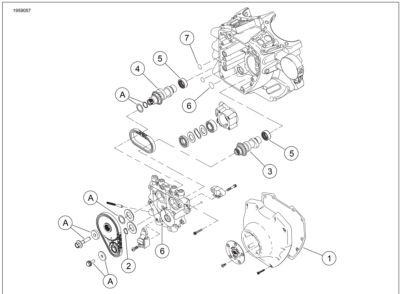
図3。交換用パーツ:Screamin' EagleProTC103CI ステージ4キット
