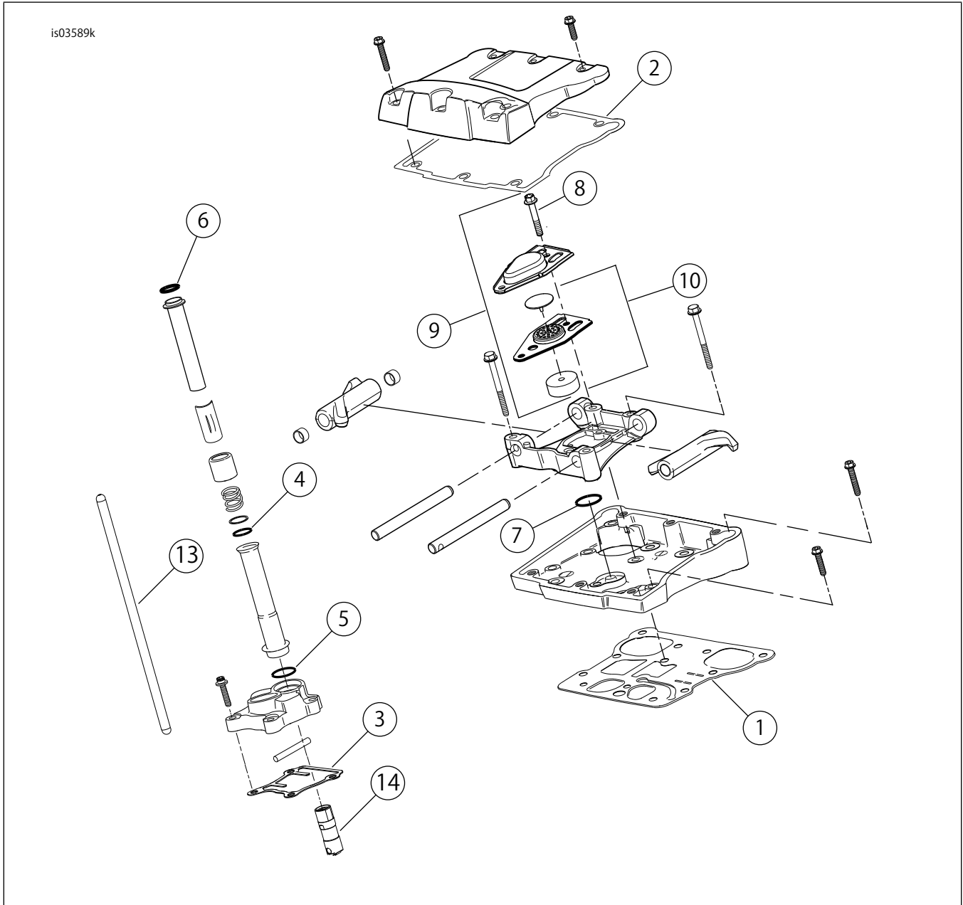
図2。交換用パーツ:Screamin' EagleProTC103CI ステージ4キット
