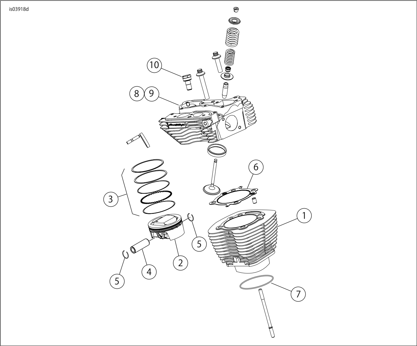
図1。交換用パーツ:Screamin' EaglePro TC 103CI ステージ4キット
