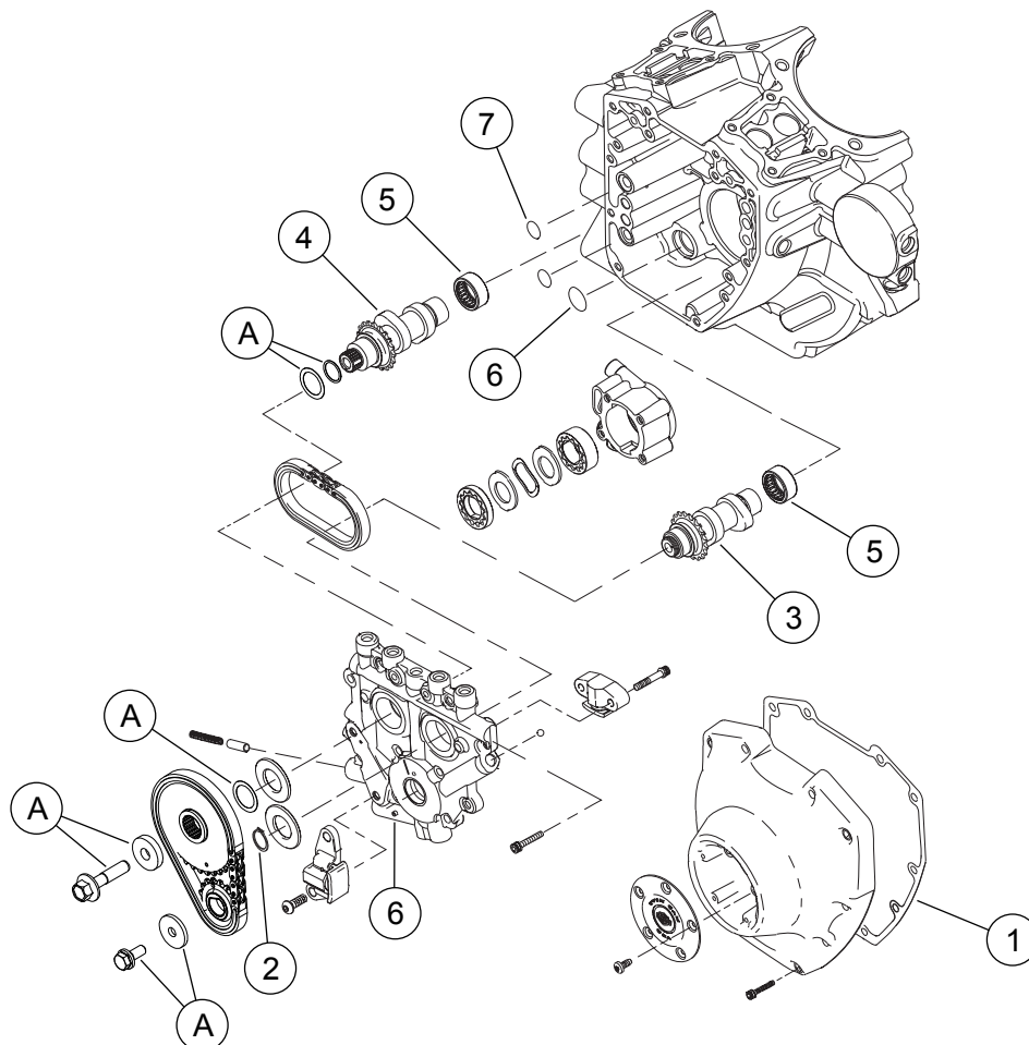
Slika 3. Servisni dijelovi: Screamin' Eagle Pro TC 103 CI Stage 4 komplet
