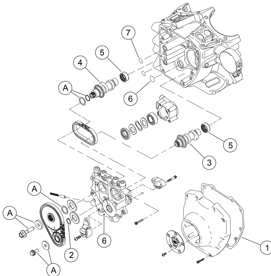
Figur 3. Reservedele: Screamin' Eagle Pro TC 103 CI Trin 4 sæt
