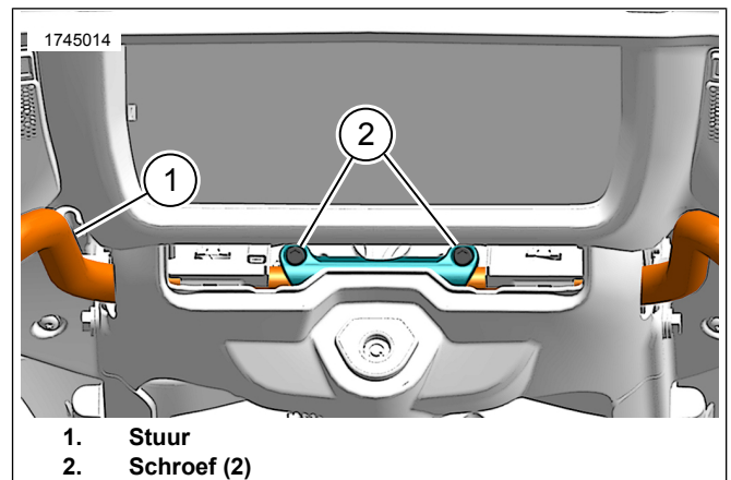
Afbeelding 2. Stuurschroef
