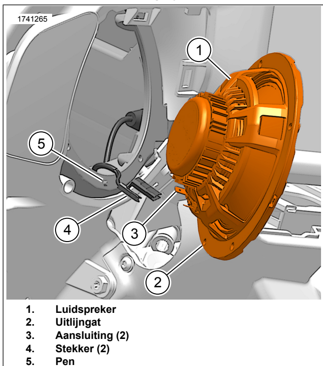
Afbeelding 4. Kuiluidspreker aansluiting
