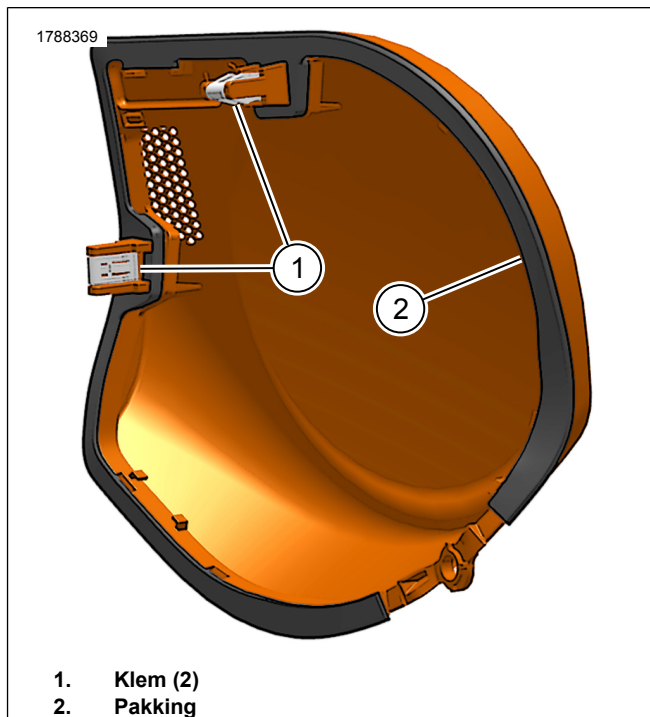
Afbeelding 6. Rooster pakking
