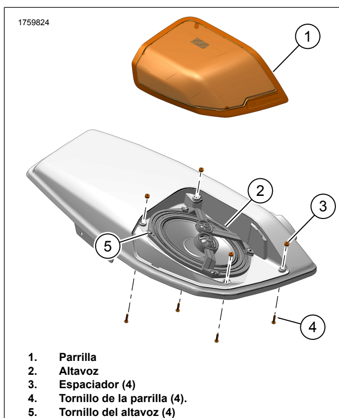
Figura 2. Conjunto de altavoces y parrilla (típico)
