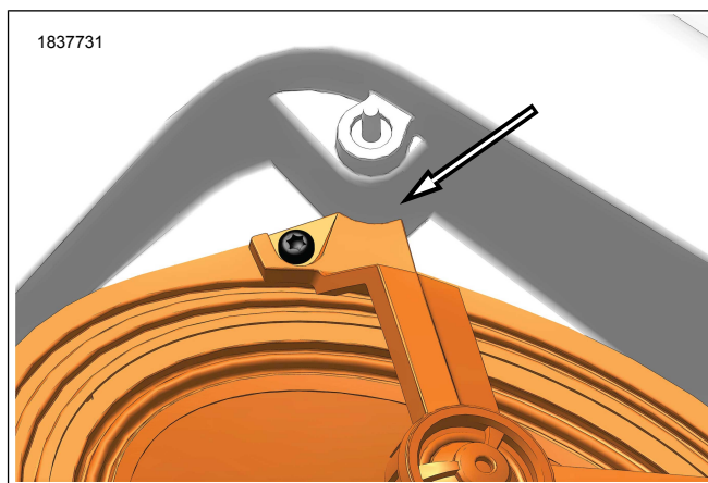
Figura 3. Orientación de la tapa del altavoz con respecto a la alforja
