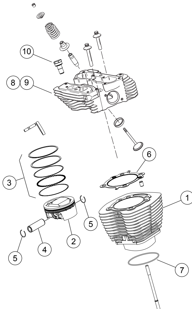
Attēls 1 Apkopes daļas: Screamin' Eagle TC 103 (1690 cc) 4. posma komplekts
