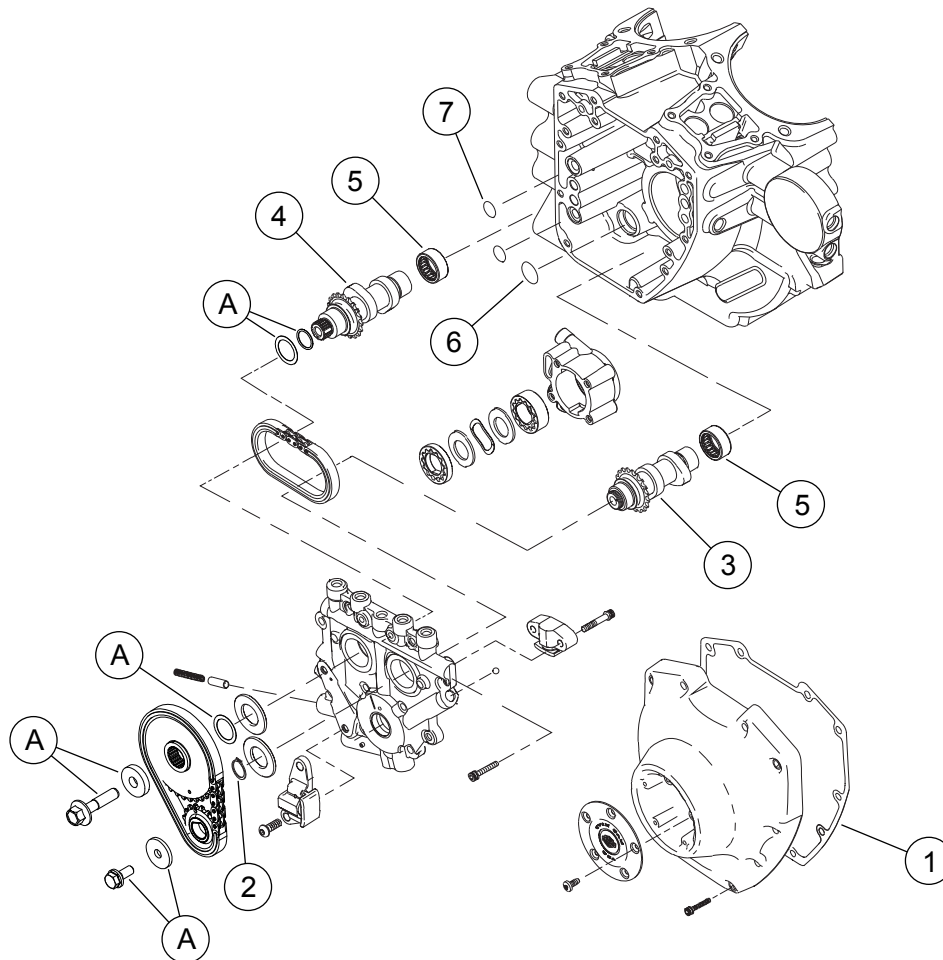
Slika 3. Servisni deli: Komplet Screamin' Eagle Pro TC 103 (1690 cc) Stage 4
