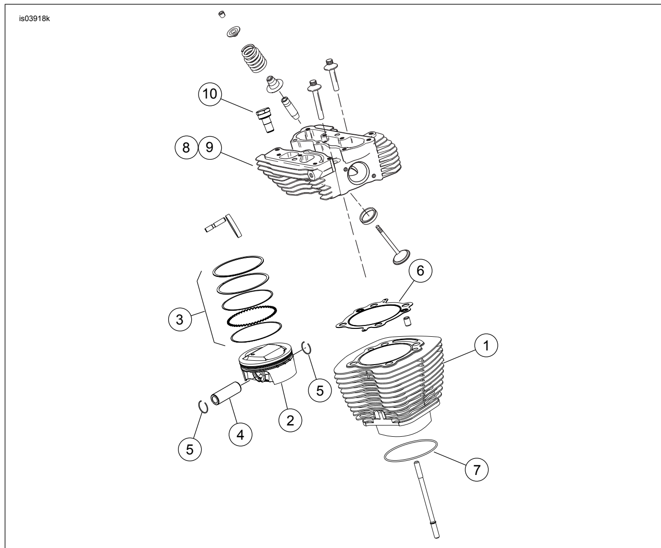
Pav 1. Dalys, reikalingos užduočiai atlikti "Screamin' Eagle" TC 103 (1690 cc) 4 etapo komplektas
