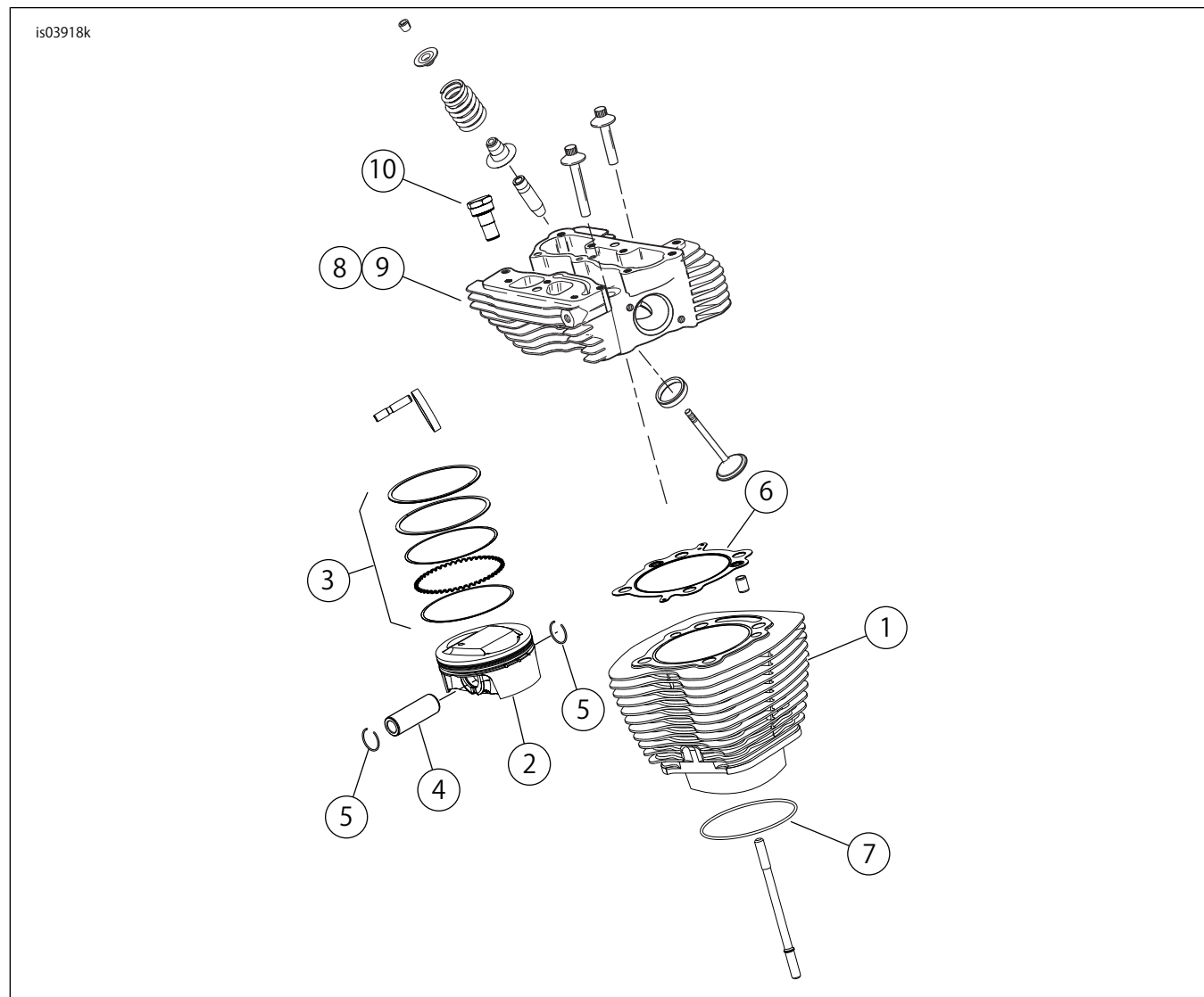
図1。交換用パーツ:Screamin' EagleTC103 (1690cc) ステージ4キット
