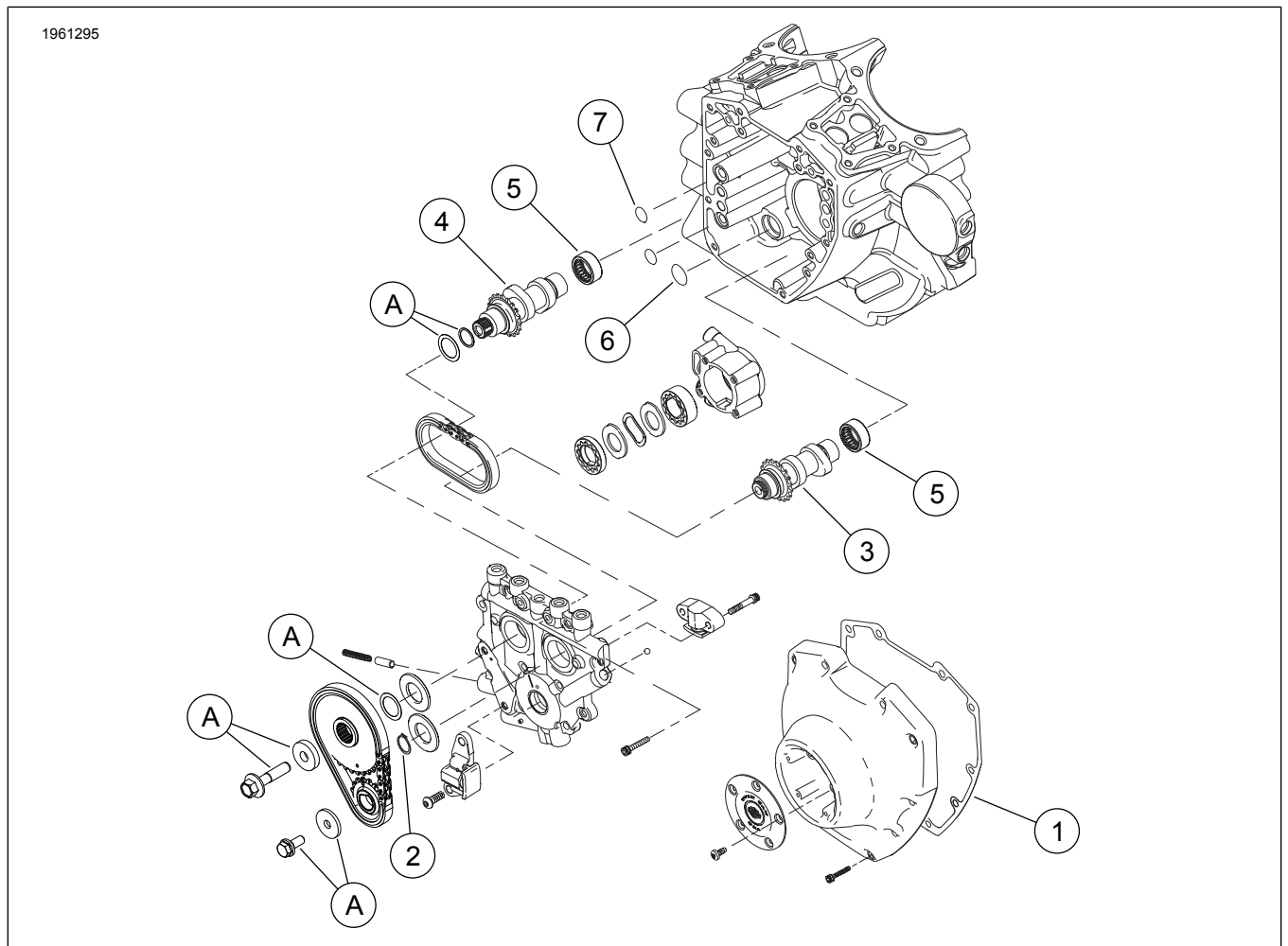
図3。交換用パーツ:Screamin' EaglePROTC103 (1690cc) ステージ4キット
