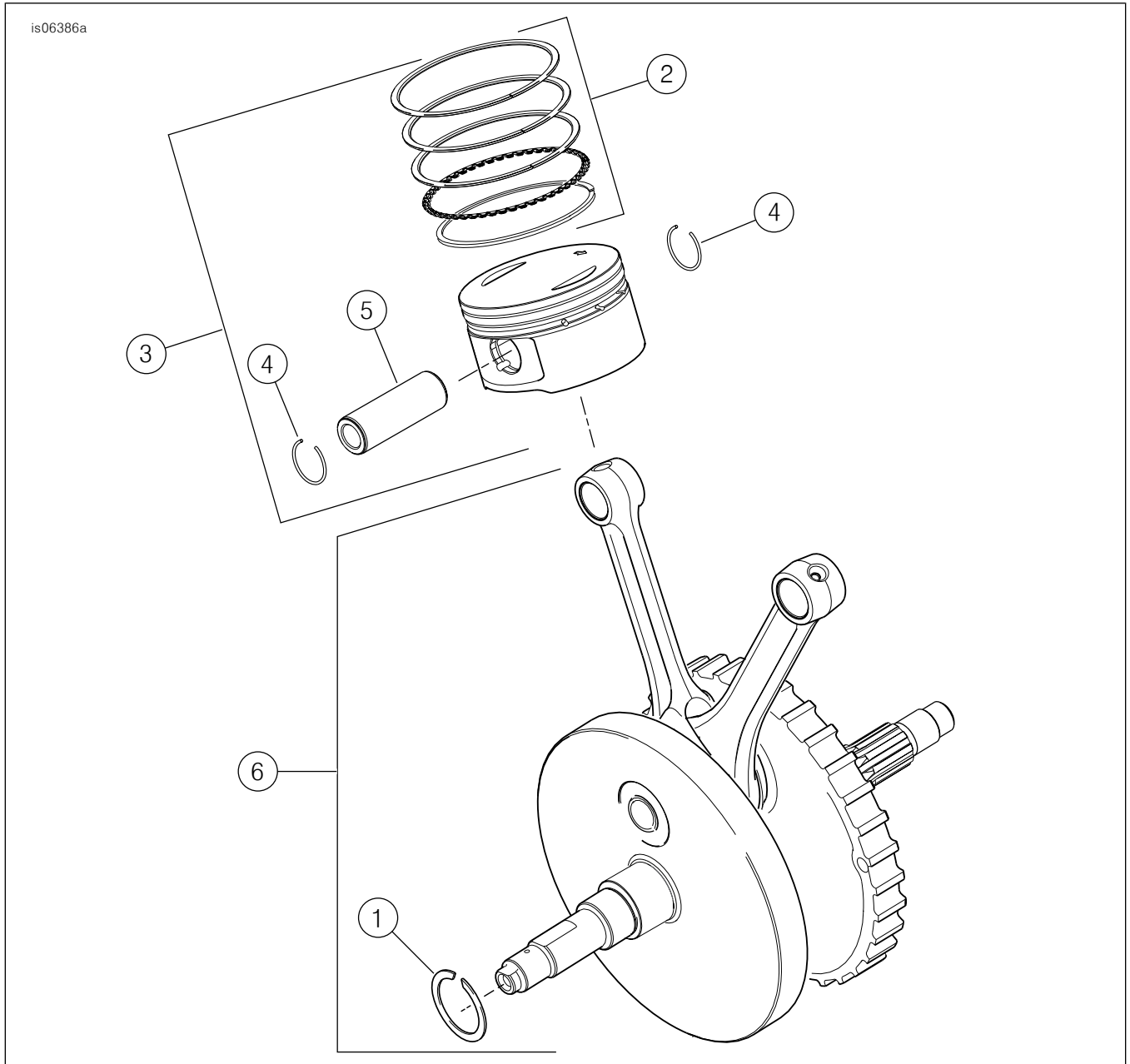
그림 11. SE120R Screamin' Eagle Pro 크레이트 엔진(베타) 피스톤 및 플라이휠
