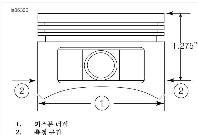
그림 2. 피스톤 측정
