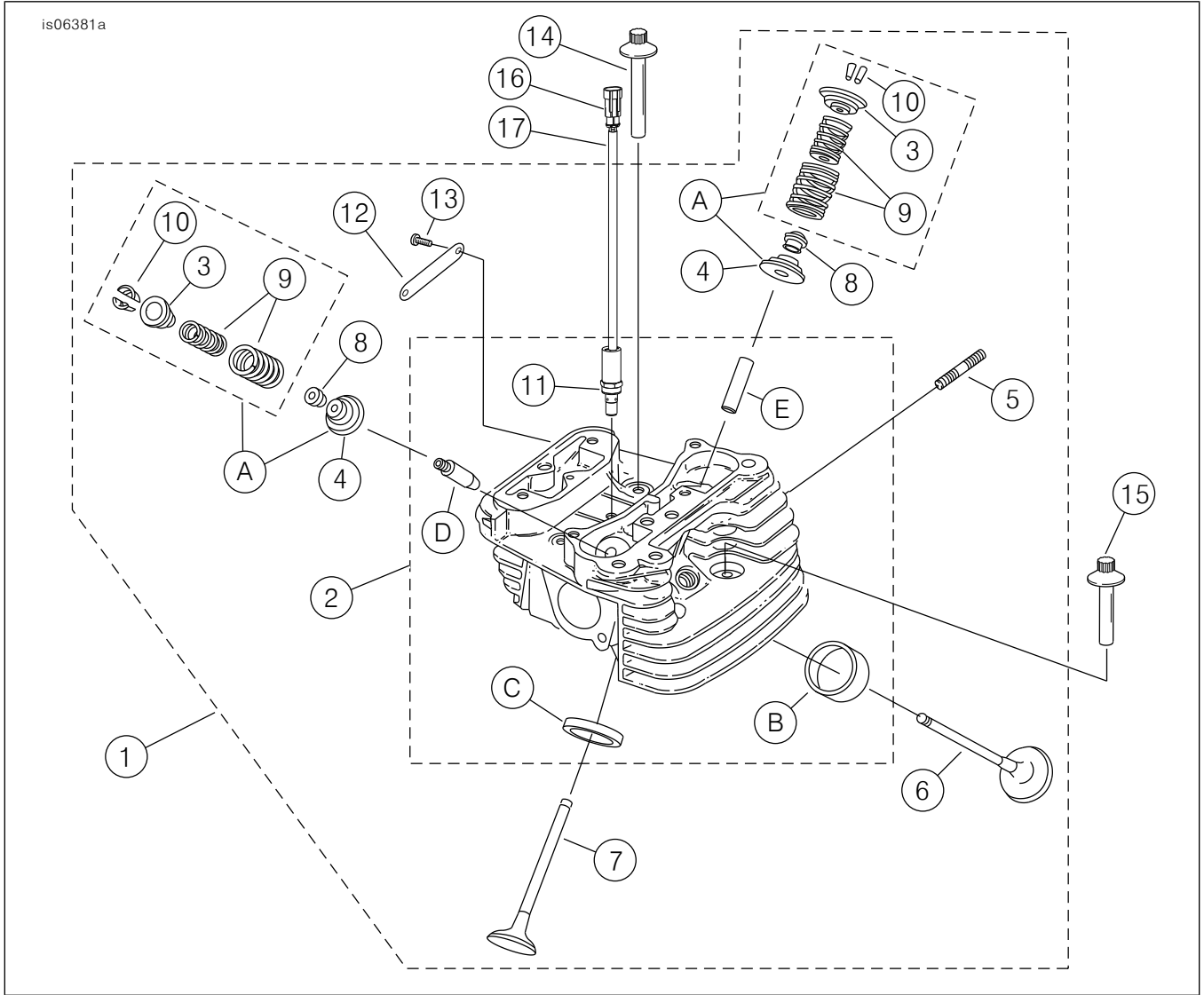
그림 9. SE120R Screamin' Eagle Pro 크레이트 엔진(베타) 실린더 헤드 및 밸브
