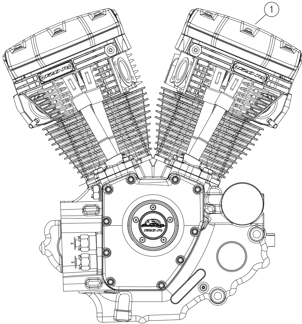
그림 7. 엔진 조립체, Screamin' Eagle Pro 120R 크레딧 엔진(베타) 전체
