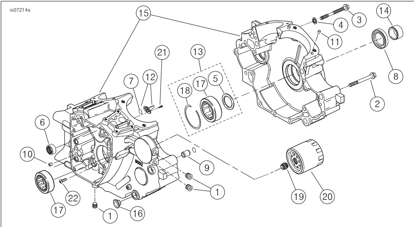
그림 12. SE120R Screamin' Eagle Pro 크레이트 엔진(베타) 크랭크케이스, 엔진 오일 필터 및 클러
