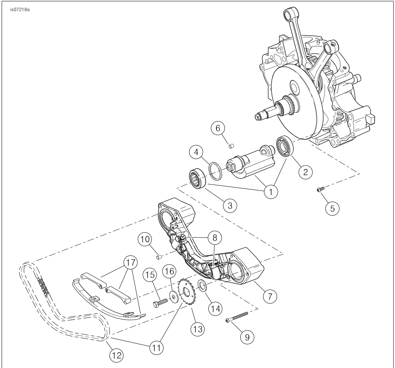
그림 13. 정비 부품: SE120R Screamin' Eagle Pro 크레이트 엔진(베타) 엔진 밸런서
