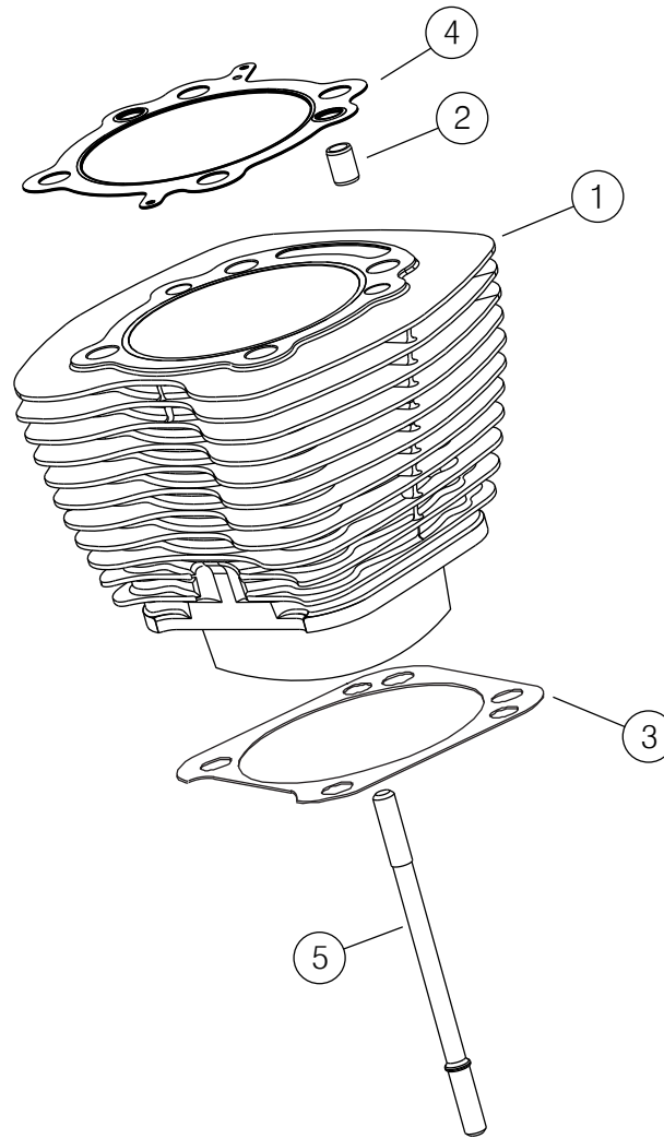
그림 8. SE120R Screamin' Eagle Pro 크레이트 엔진(베타) 실린더
