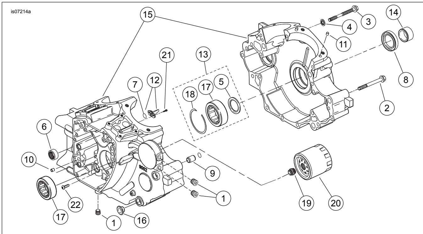
Hình 12. Các-te Động cơ thùng SE120R Screamin' Eagle Pro (Beta), Bộ lọc dầu động cơ và bộ làm mát
