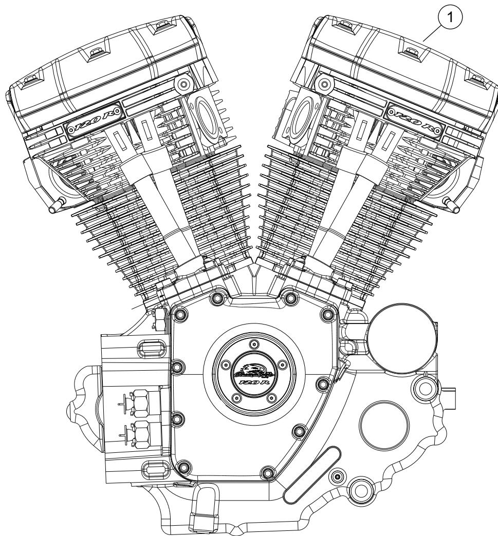
Hình 7. Cụm động cơ, Screamin' Eagle Pro 120R Crate Engine (Beta) Hoàn thành
