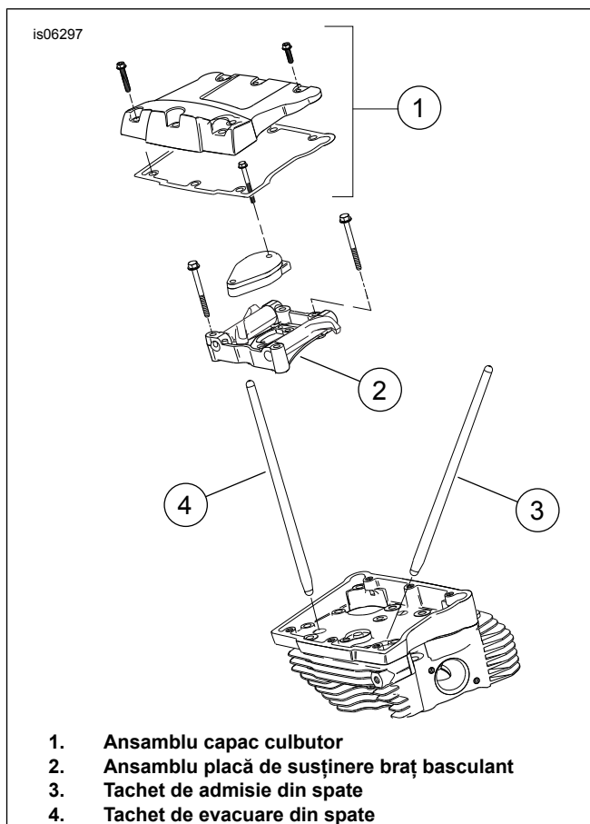
Figura 6. Tacheți
