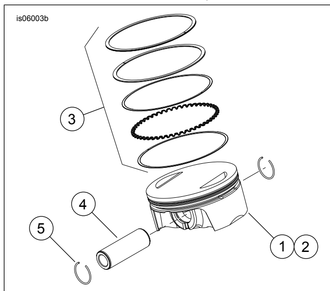
Figura 5. Ansamblul pistonului
