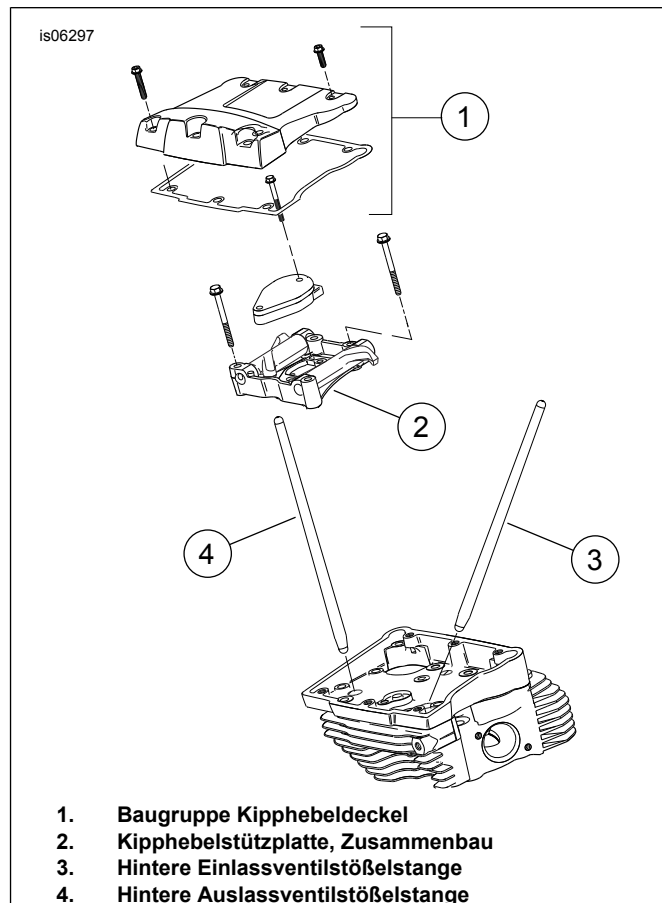
Abbildung 6. Stößelstangen
