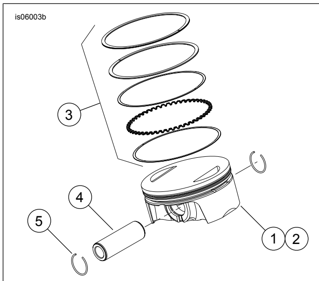
Abbildung 5. Kolben-Baugruppe
