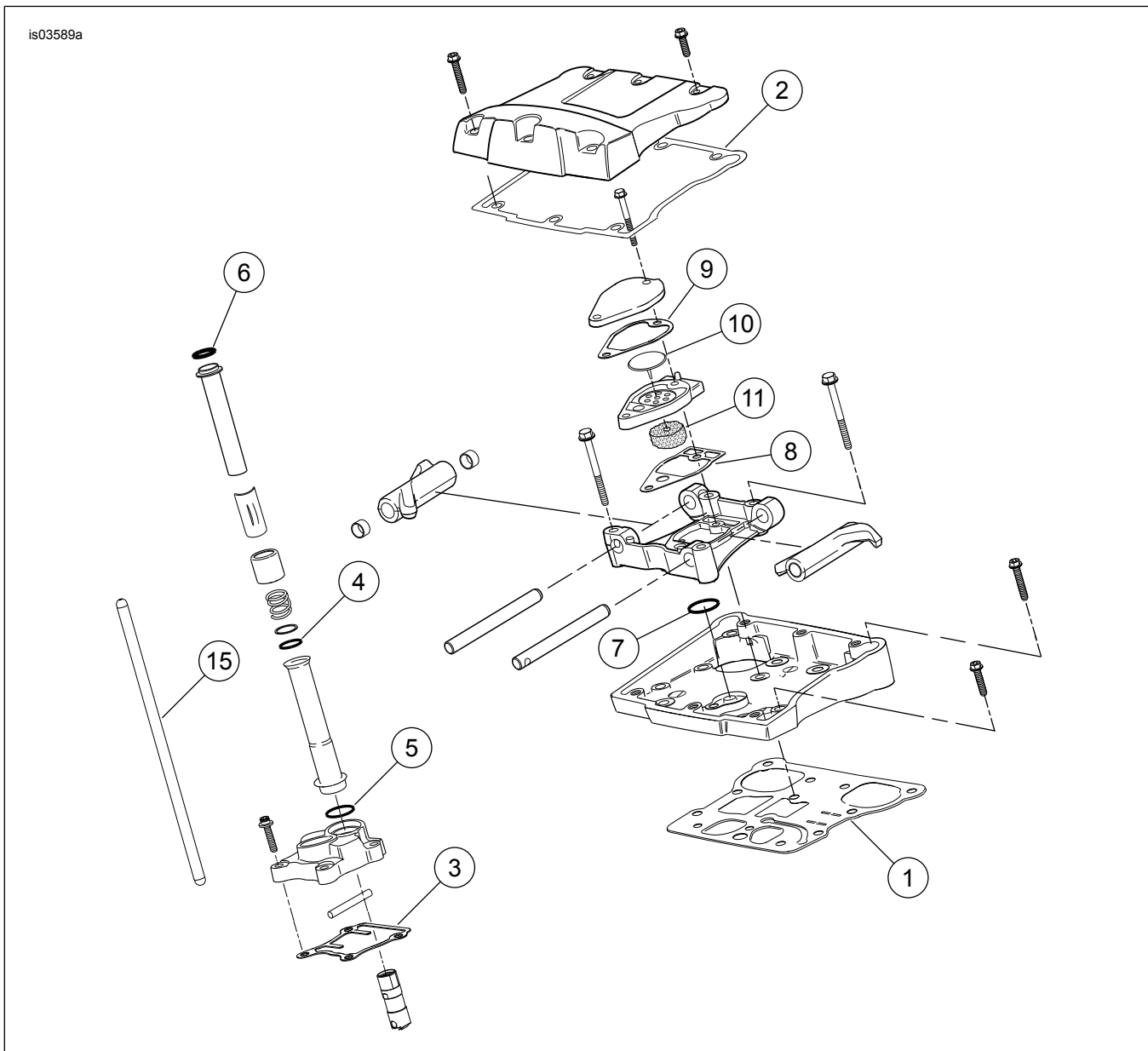
Figure 2. Mga Pamalit na Piyesa: Screamin' Eagle Pro TC 103 (1690 cc) Stage 4 Kit
