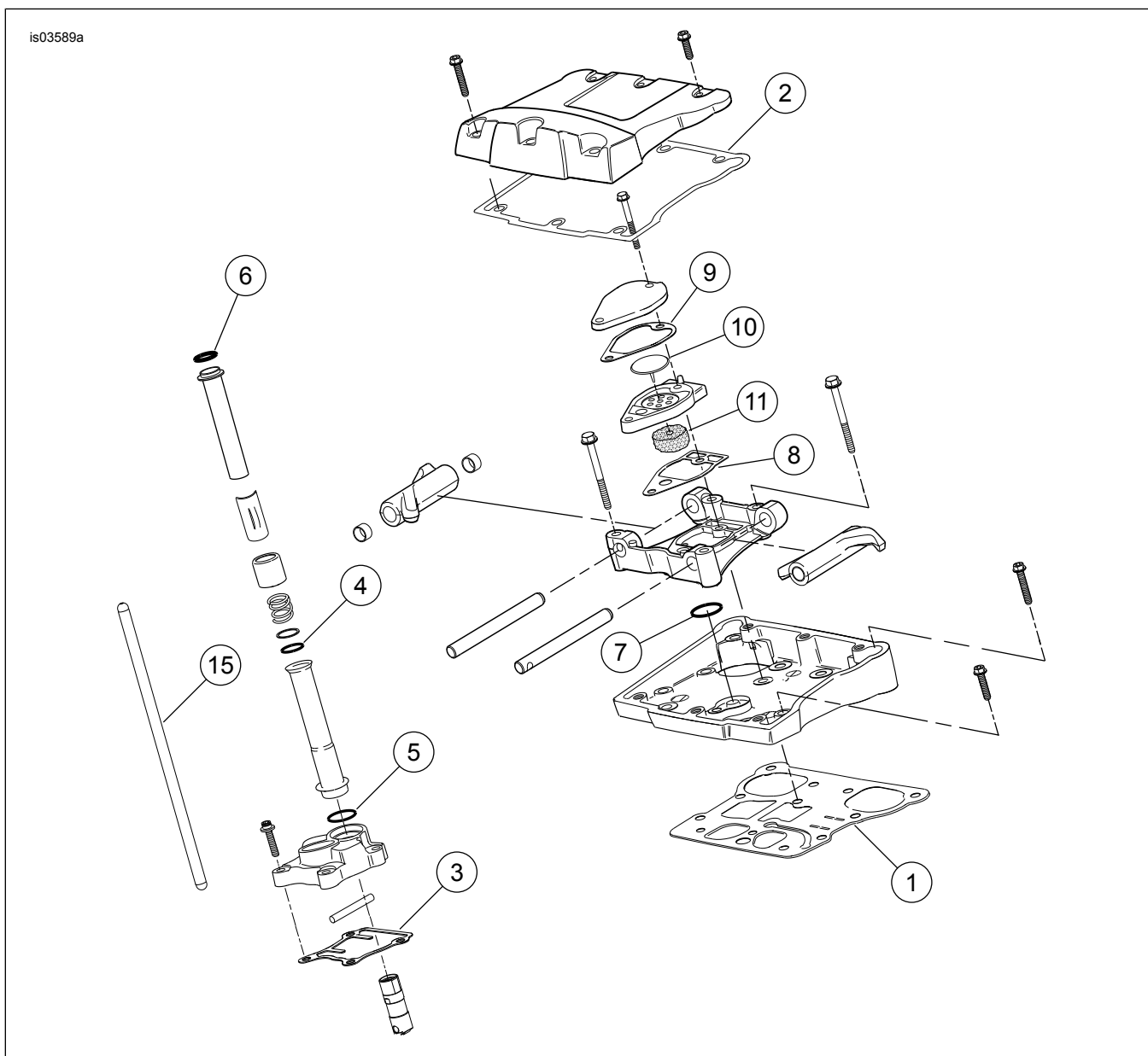
Figura 2. Componente de service: Kit Etapa 4 Screamin' Eagle Pro TC 103 (1690 cc)
