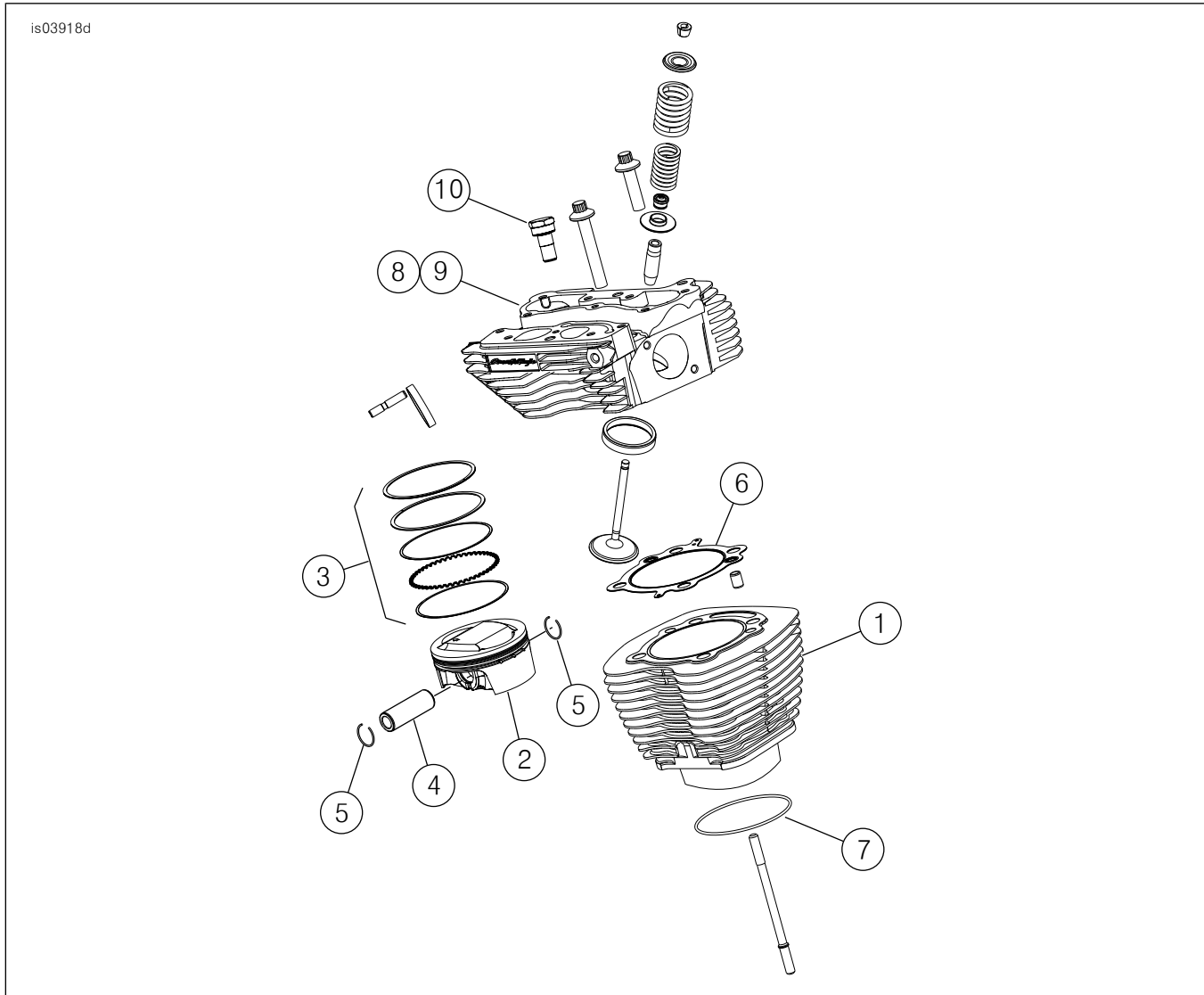
그림 1. 정비 부품: Screamin' Eagle Pro TC 103(1690cc) 스테이지 4 키트
