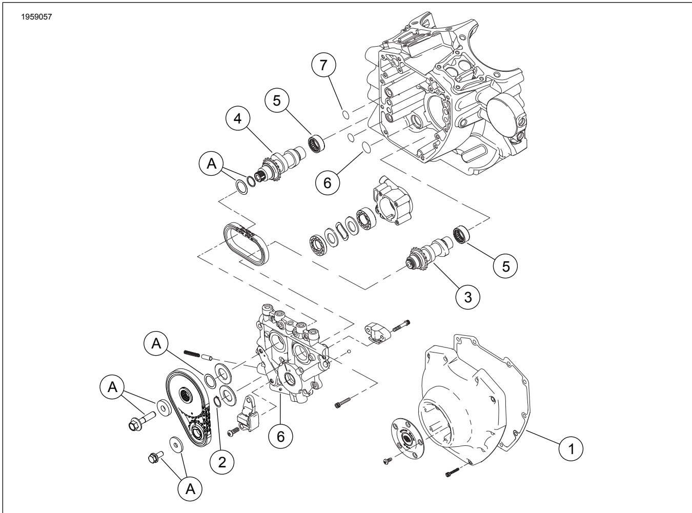
그림 3. 정비 부품: Screamin' Eagle Pro TC 103(1690cc) 스테이지 4 키트
