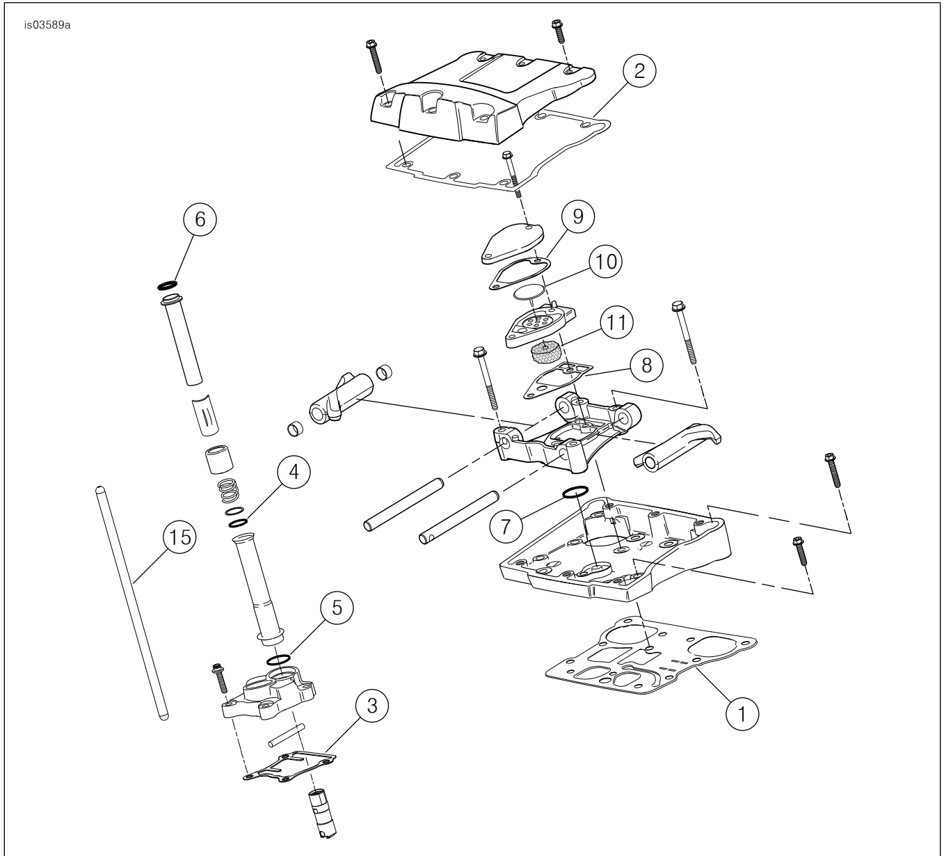
그림 2. 정비 부품: Screamin' Eagle Pro TC 103(1690cc) 스테이지 4 키트
