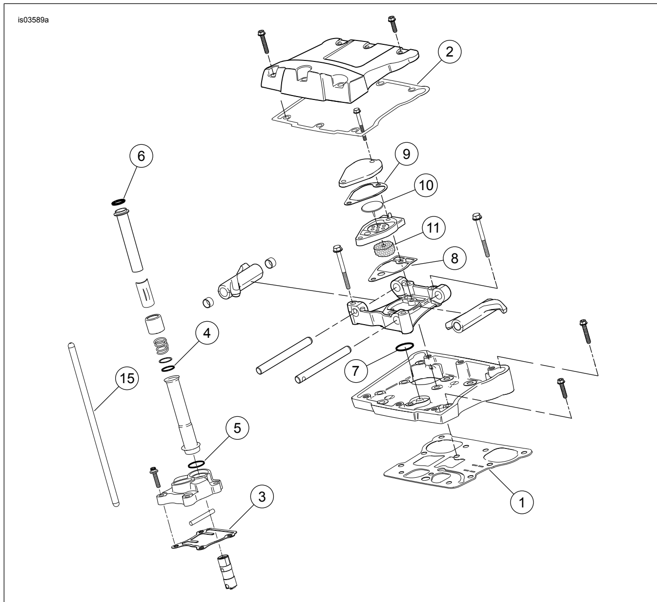
Slika 2. Servisni deli: Komplet Screamin' Eagle Pro TC 103 (1690 cc) Stage 4
