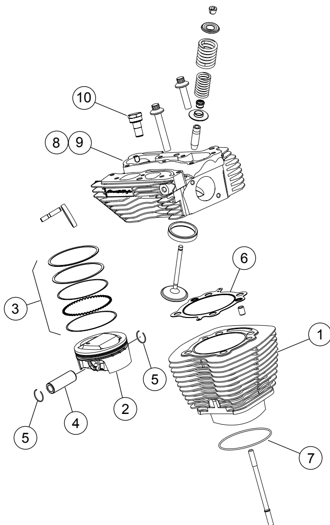
Slika 1. Servisni deli: Komplet Screamin' Eagle Pro TC 103 (1690 cc) Stage 4
