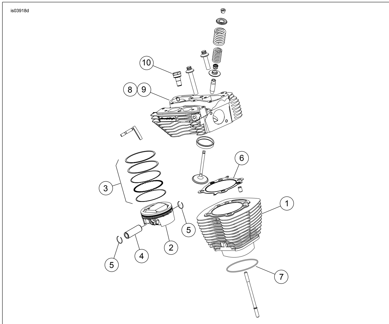
Pav 1. Dalys, reikalingos užduočiai atlikti "Screamin' Eagle Pro" TC 103 (1690 cc) 4 etapo komplektas
