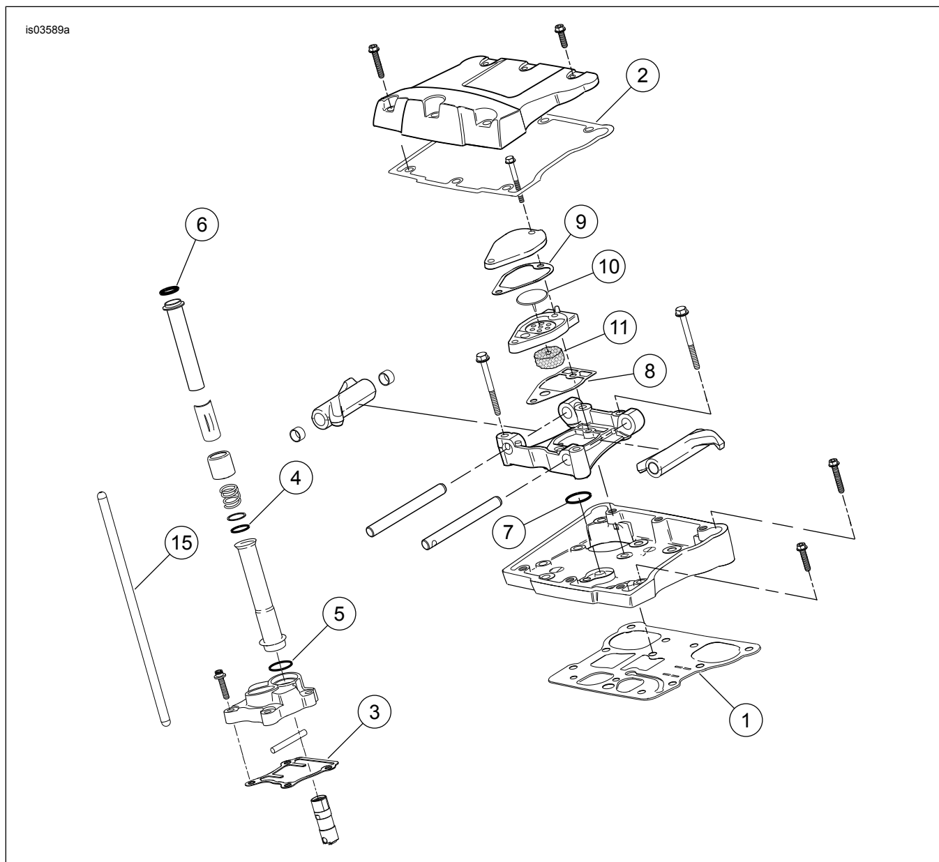
Pav 2. Dalys, reikalingos užduočiai atlikti "Screamin' Eagle Pro" TC 103 (1690 cc) 4 etapo komplektas
