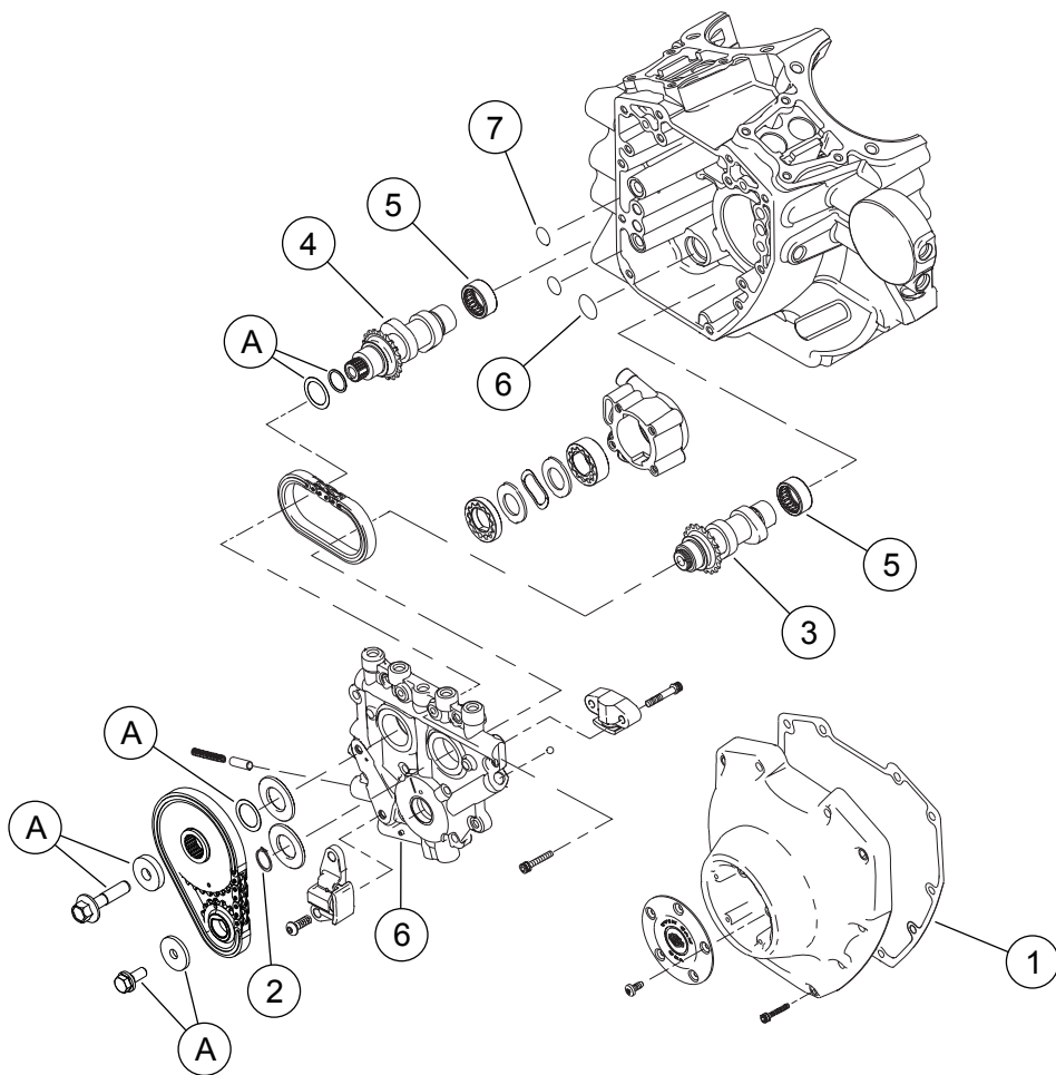
Pav 3. Dalys, reikalingos užduočiai atlikti "Screamin' Eagle Pro" TC 103 (1690 cc) 4 etapo komplektas
