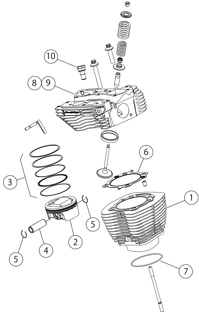
図1。交換用パーツ:Screamin' EaglePRO TC103 (1690 cc) ステージ4キット
