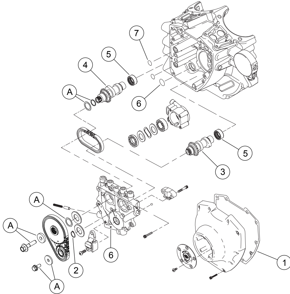
図3。交換用パーツ:Screamin' EaglePROTC103 (1690cc) ステージ4キット
