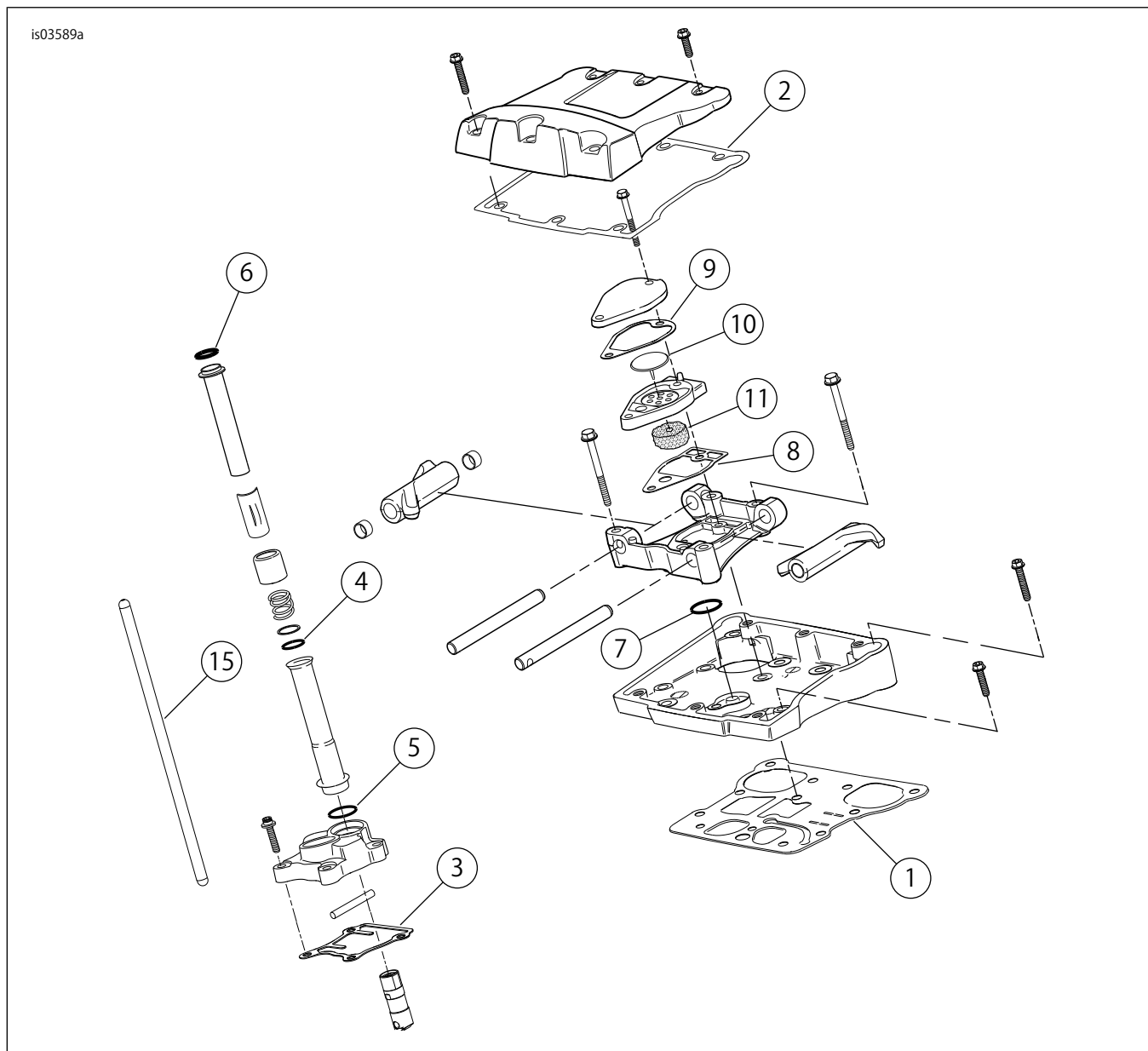
図2。交換用パーツ:Screamin' EaglePROTC103 (1690cc) ステージ4キット
