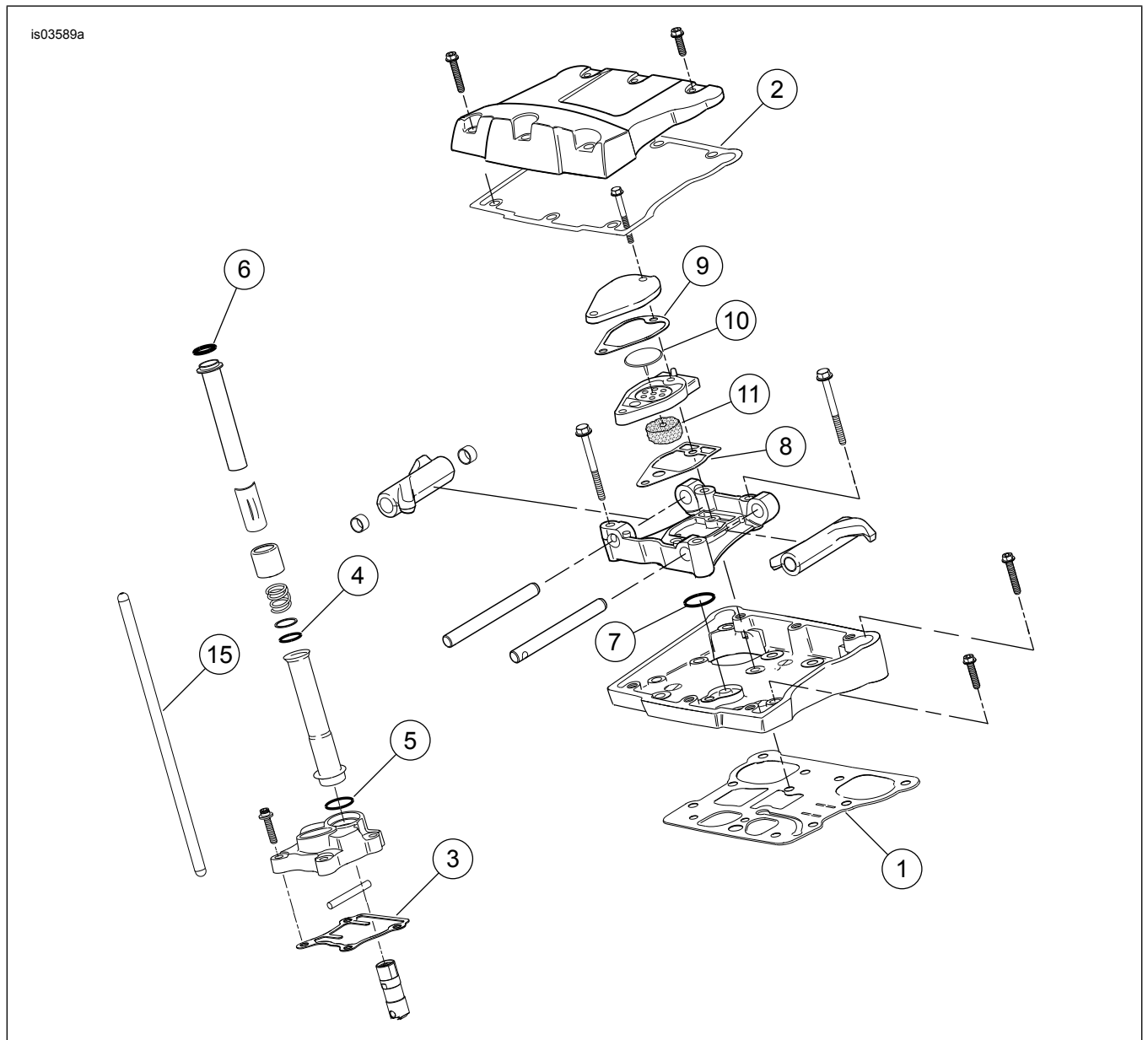
Afbeelding 2. Serviceonderdelen: Screamin' Eagle Pro TC 1690 cm 3 (103) Stage 4-set
