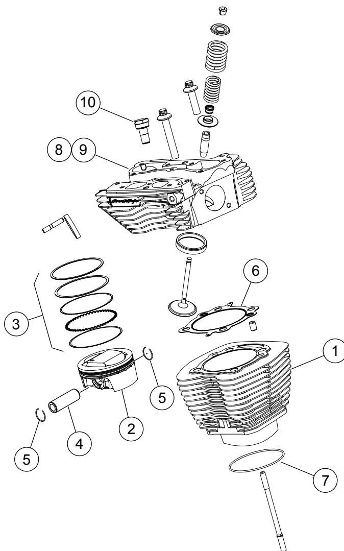
Afbeelding 1. Serviceonderdelen: Screamin' Eagle Pro TC 1690 cm³ (103) Stage 4-set
