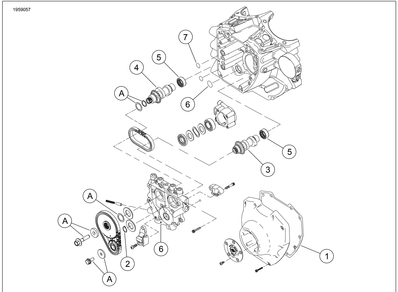
Figure 3. Mga Pamalit na Piyesa: Screamin' Eagle Pro TC (96 ci hanggang 103 ci) Stage 4 Kit
