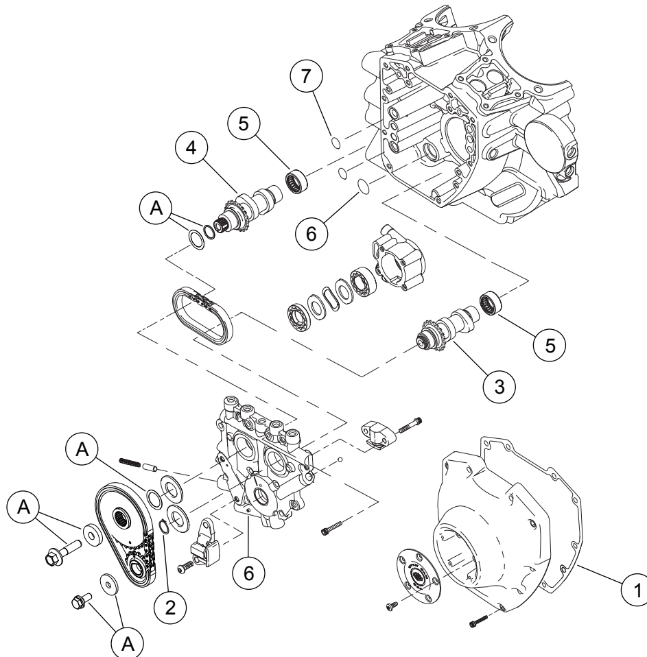
Ábra 3. Szervizelhető alkatrészek: Screamin' Eagle Pro TC 103 (96 ci – 103 ci) Stage 4. készlet
