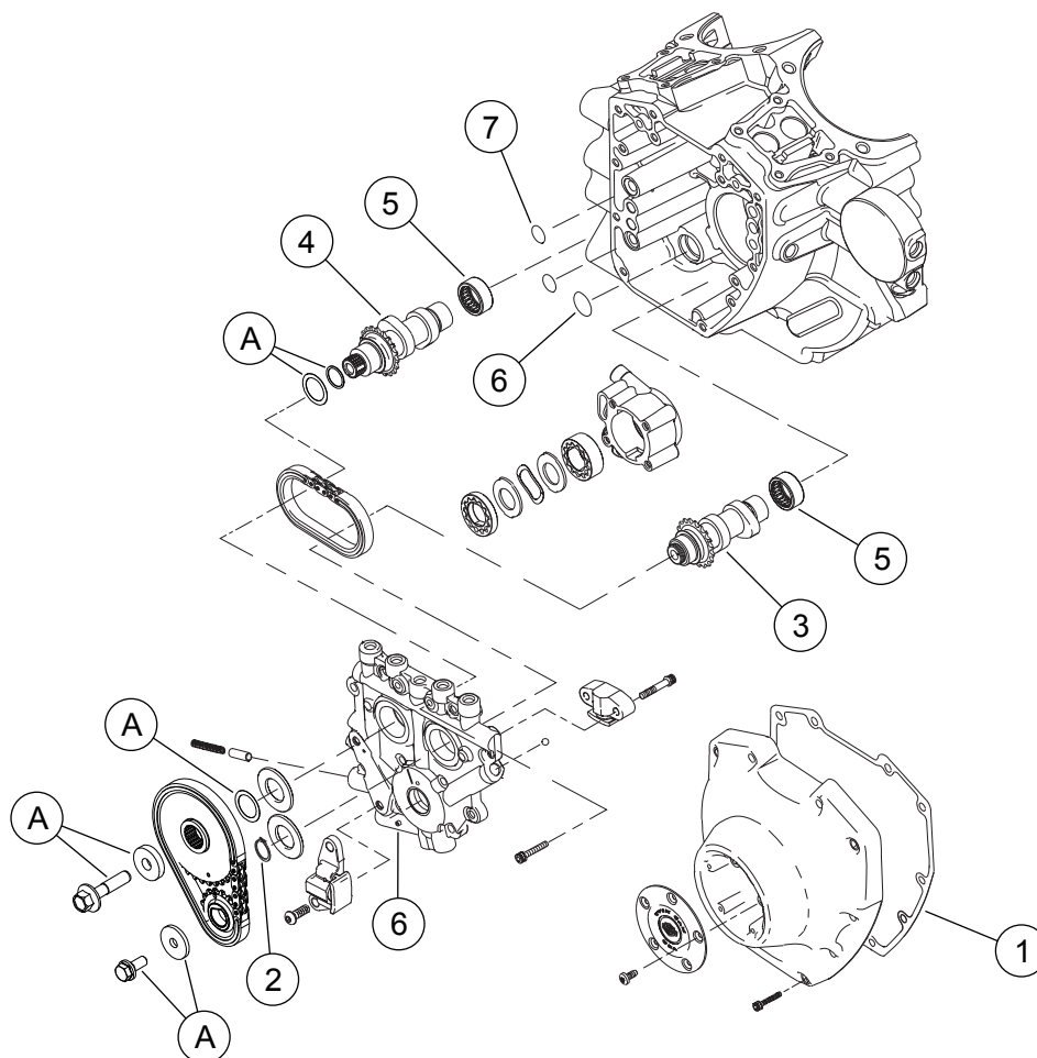
Attēls 3 Apkopes daļas: Screamin' Eagle Pro TC (96 ci līdz 103 ci) 4. posma komplekts
