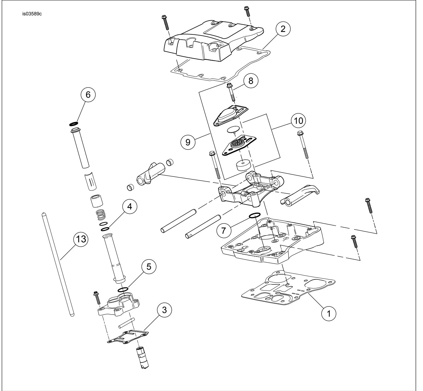
Şekil 2. Servis Parçaları: Screamin' Eagle Pro TC (96 ci - 103 ci) Stage 4 Kiti
