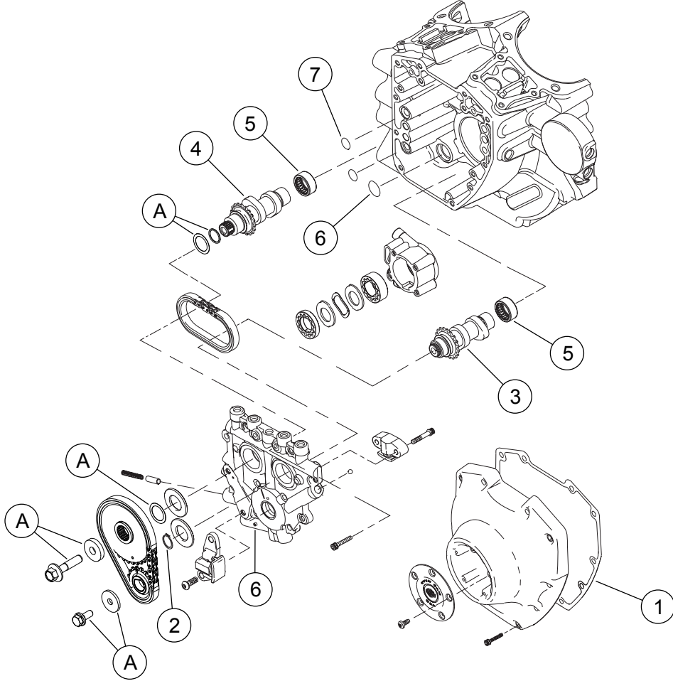
Şekil 3. Servis Parçaları: Screamin' Eagle Pro TC (96 ci - 103 ci) Stage 4 Kiti
