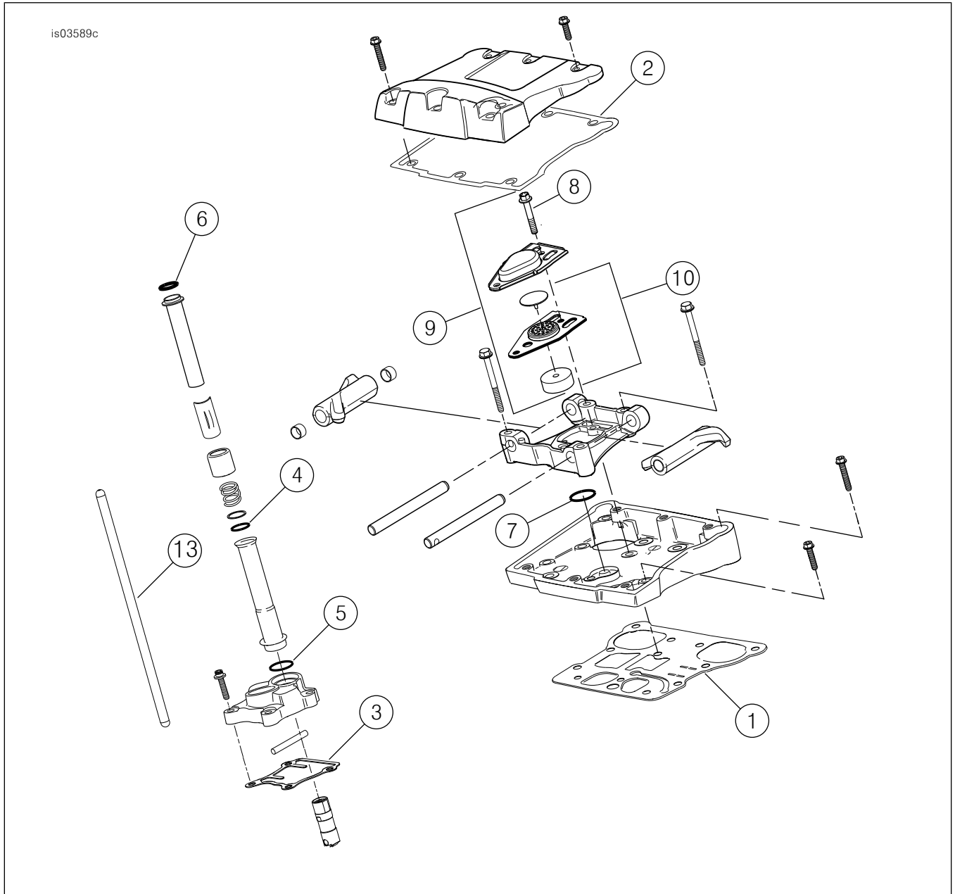
그림 2. 정비 부품: Screamin' Eagle Pro TC (96 CI ~ 103 CI) 스테이지 4 키트
