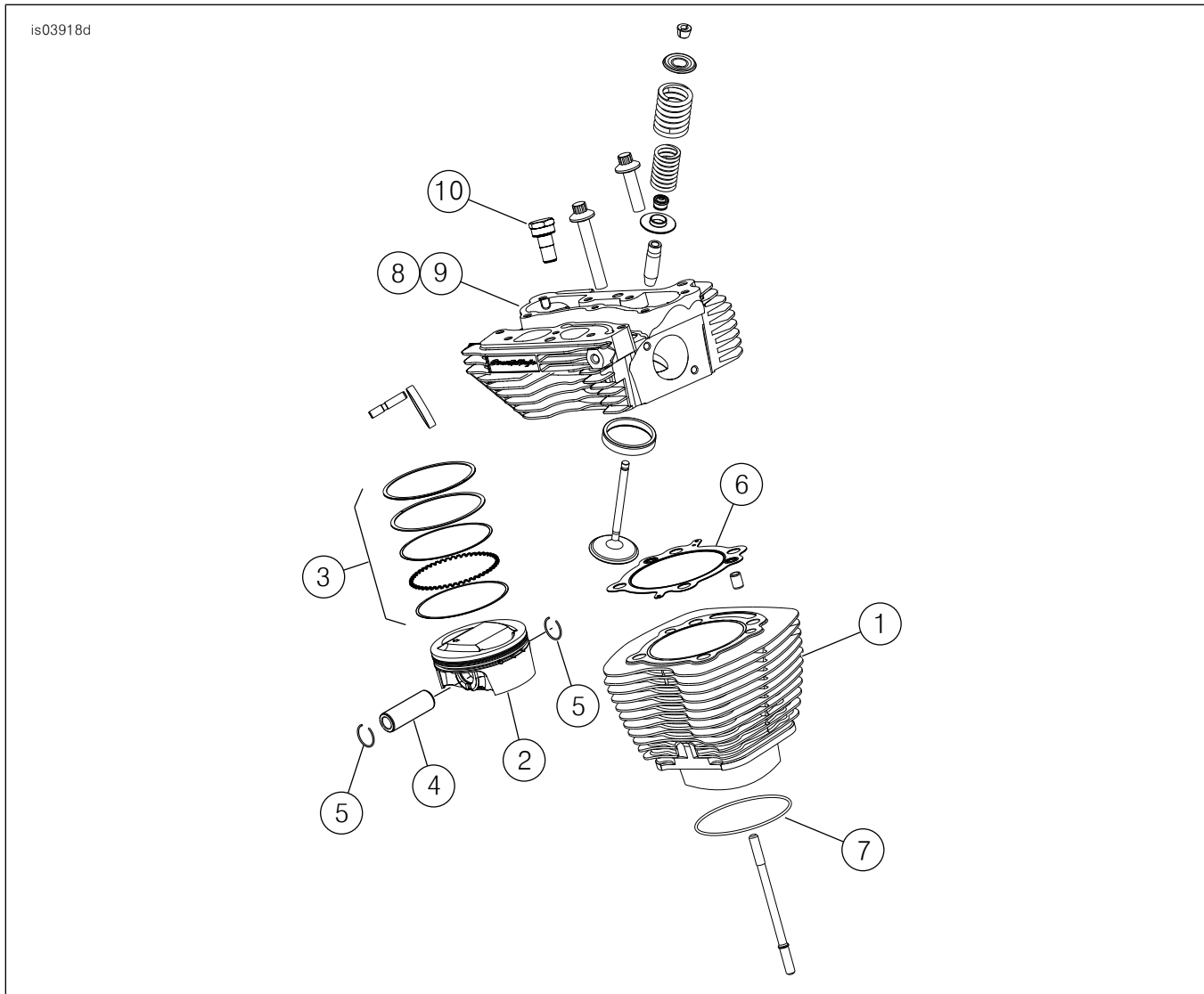
그림 1. 정비 부품: Screamin' Eagle Pro TC (96 CI ~ 103 CI) 스테이지 4 키트
