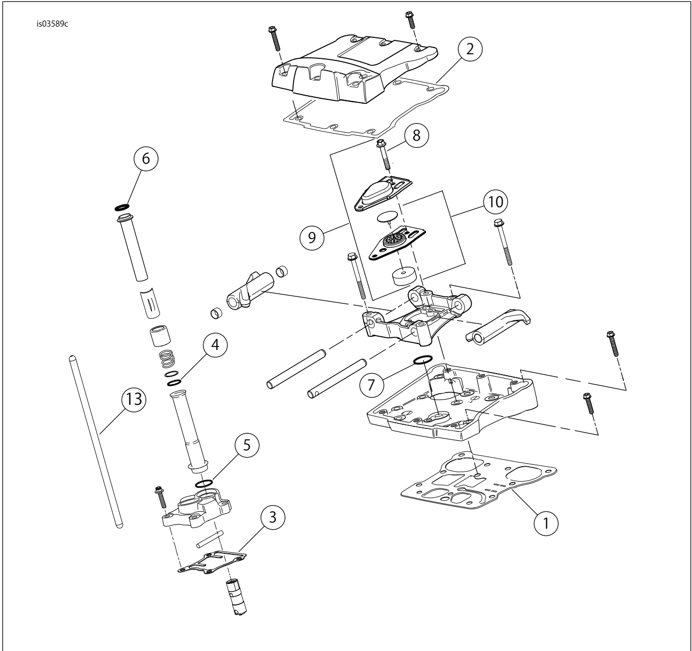
図2。交換用パーツ:Screamin' EagleProTC (96ci→103ci) ステージ4キット
