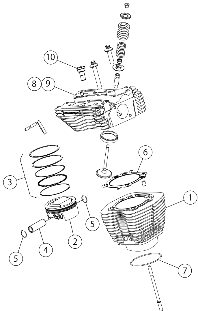
図1。交換用パーツ:Screamin' EagleProTC (96ci→103ci) ステージ4キット
