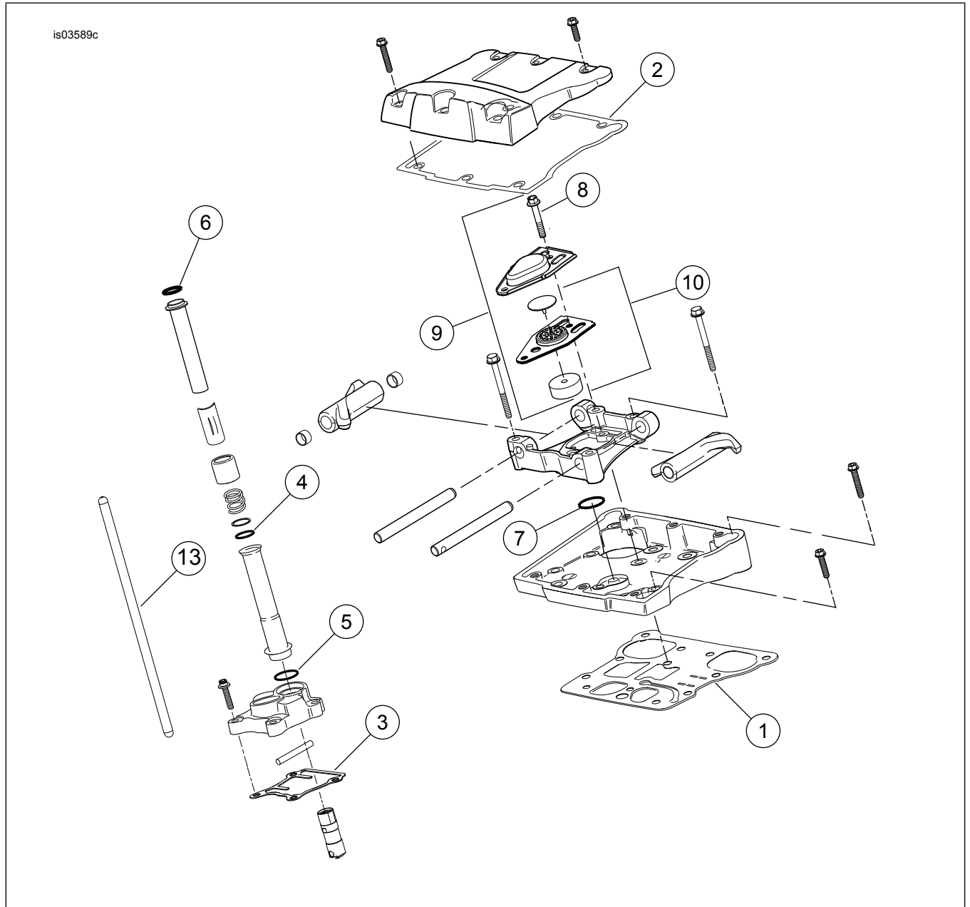
Slika 2. Servisni dijelovi: Screamin' Eagle Pro TC (96 ci do 103 ci) komplet Stage 4
