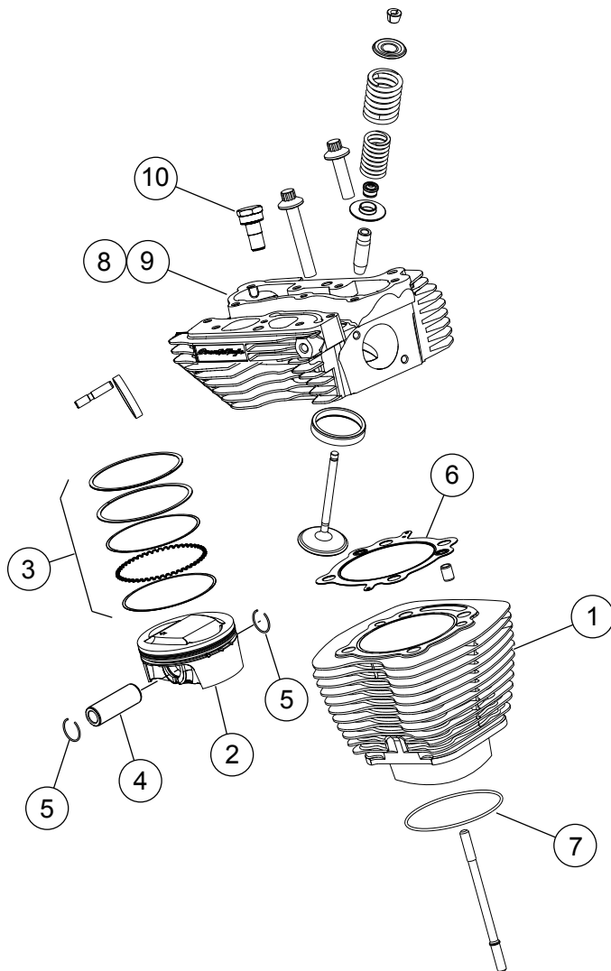
Slika 1. Servisni dijelovi: Screamin' Eagle Pro TC (96 ci do 103 ci) komplet Stage 4
