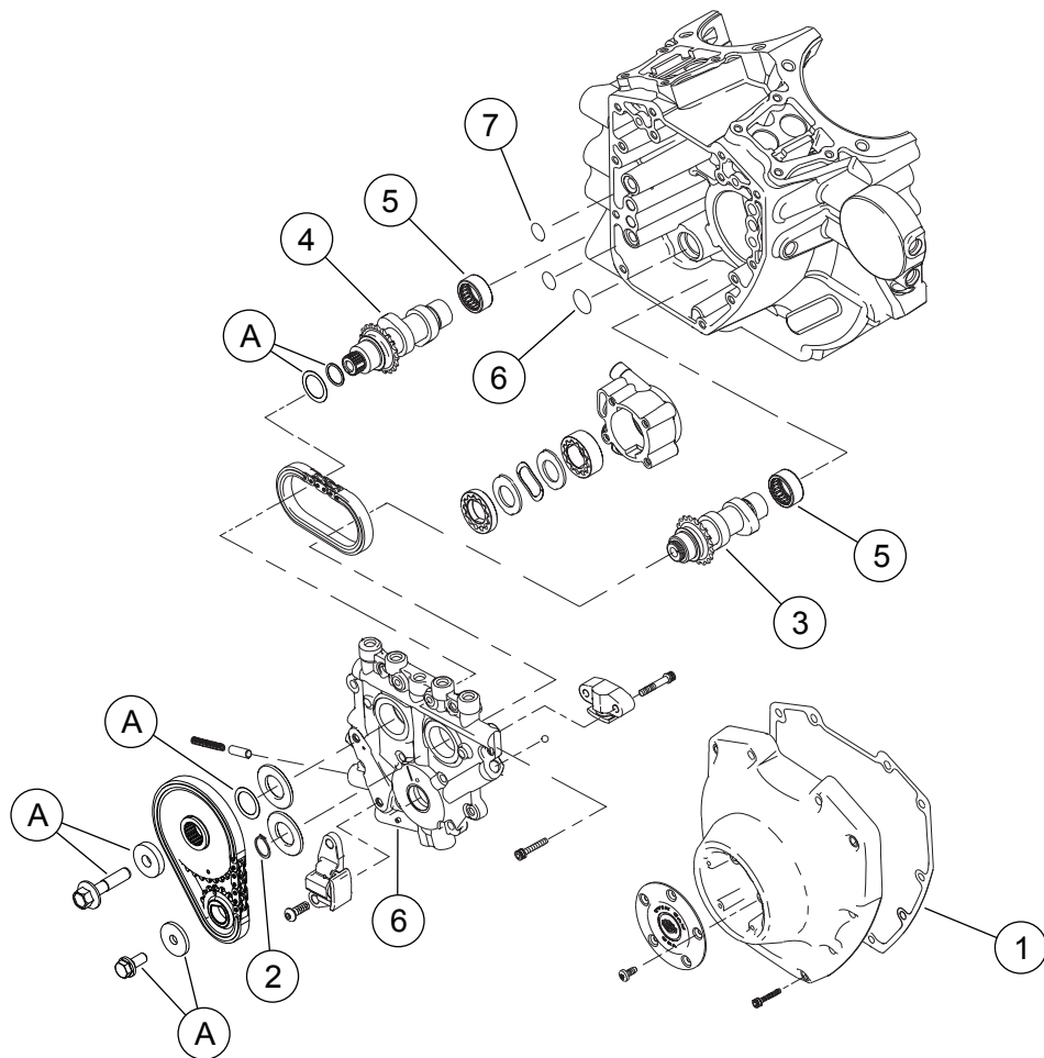
Slika 3. Servisni dijelovi: Screamin' Eagle Pro TC (96 ci do 103 ci) komplet Stage 4
