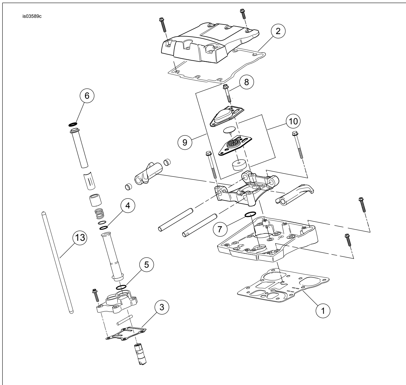
Figur 2. Reservedele: Screamin' Eagle Pro TC (96 ci til 103 ci) Stage 4 sæt
