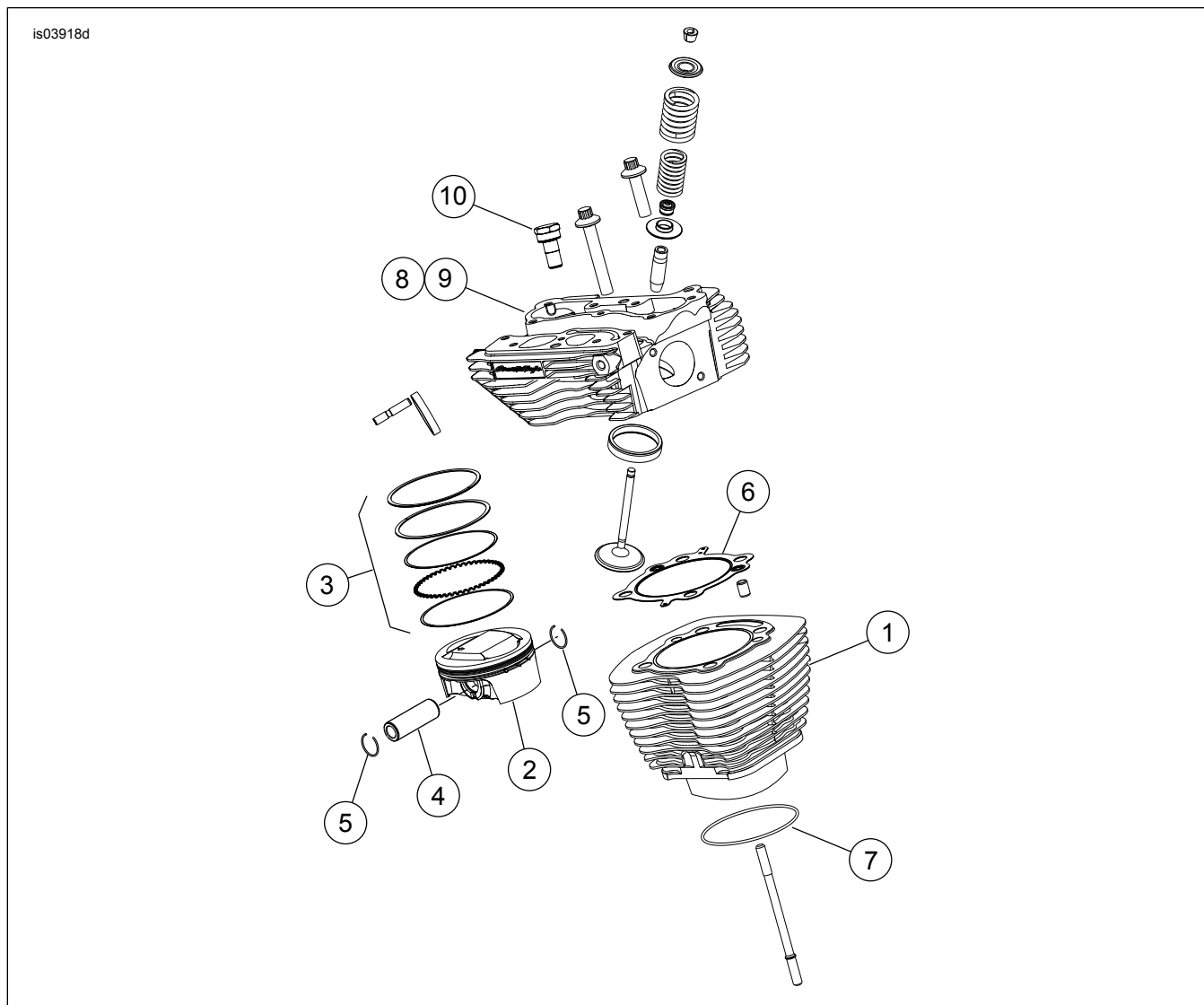
Figur 1. Reservedele: Screamin' Eagle Pro TC (96 ci til 103 ci) Stage 4 sæt
