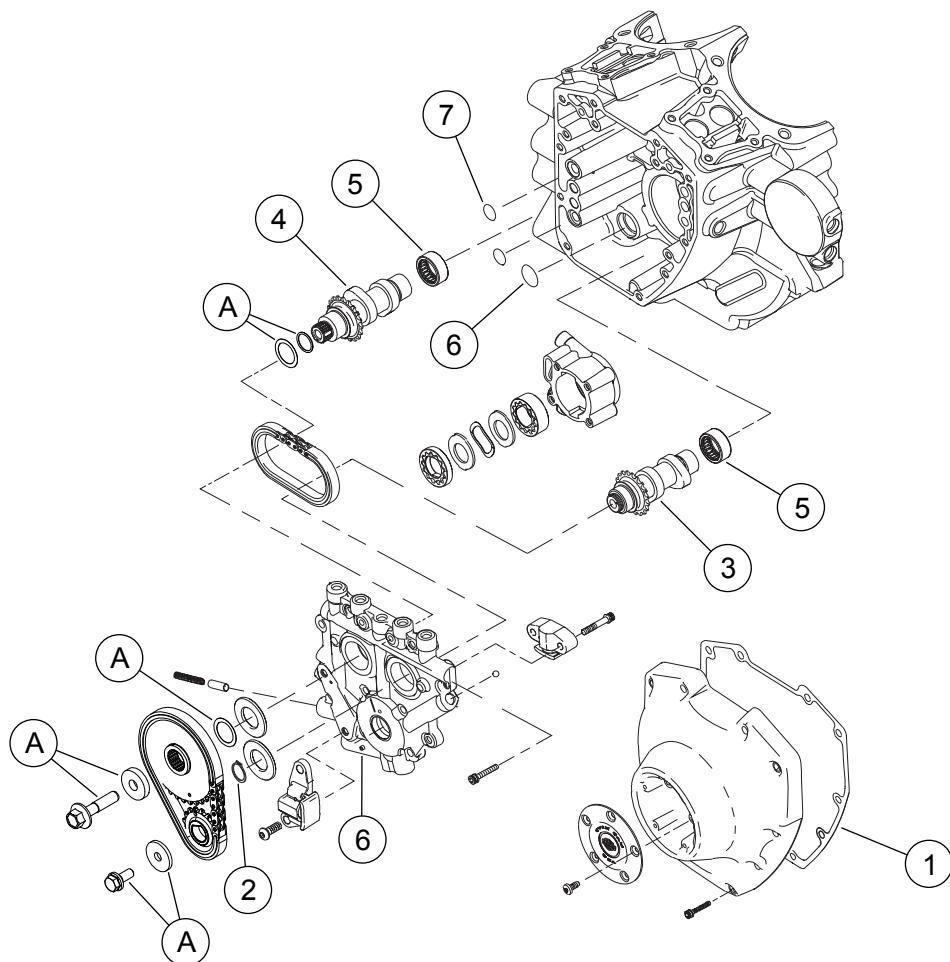
Figur 3. Reservedele: Screamin' Eagle Pro TC (96 ci til 103 ci) Stage 4 sæt
