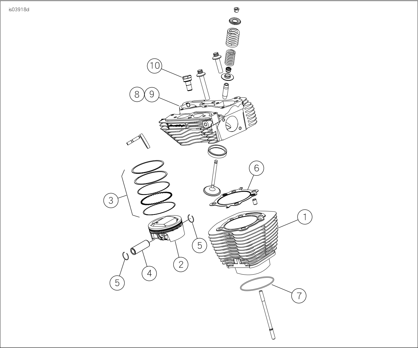
圖1。維修零件Screamin’ EagleProTC( 96ci至103ci )Stage4工具包
