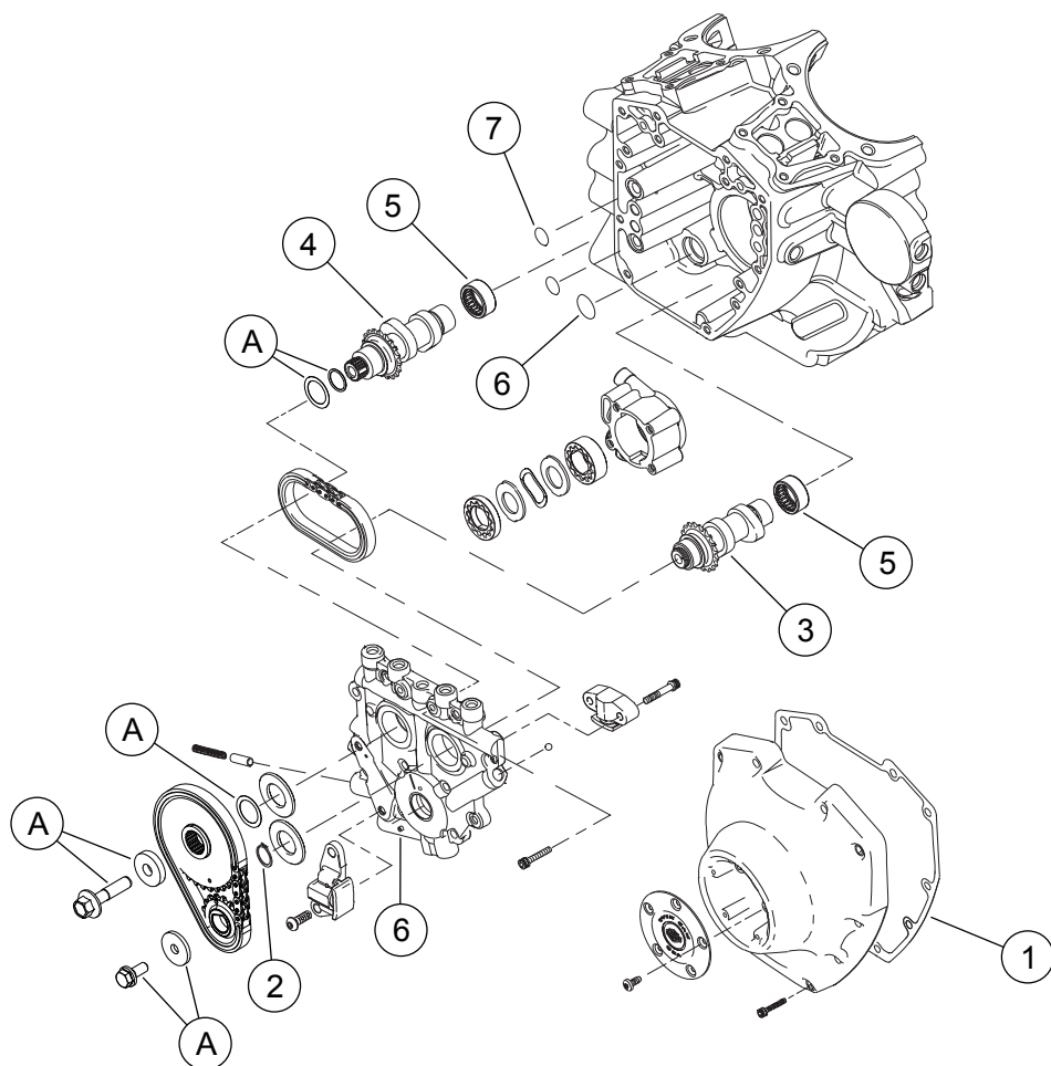
圖3。維修零件Screamin' Eagle Pro TC( 96ci 至 103ci )Stage 4工具包
