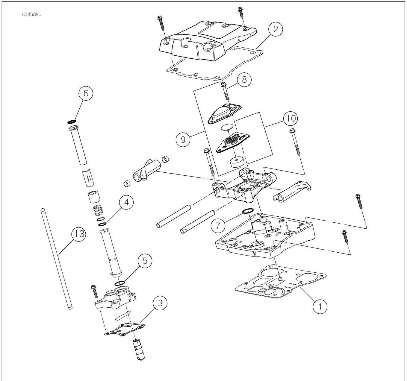
圖2。維修零件Screamin' EagleProTC( 96ci 至 103ci )Stage4工具包
