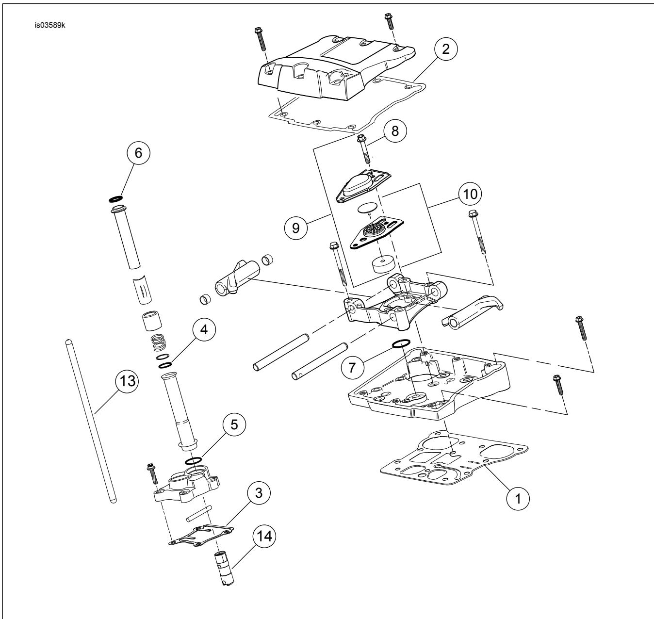
Figure 2. Mga Pamalit na Piyesa: Screamin' Eagle TC 103 (1690 cc) Stage 4 Kit
