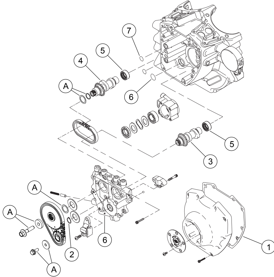
Şekil 3. Servis Parçaları: Screamin' Eagle Pro 103 (1690 cc) Stage 4 Kiti
