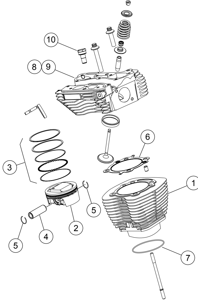
Şekil 1. Servis Parçaları: Screamin' Eagle TC 103 (1690 cc) Stage 4 Kiti
