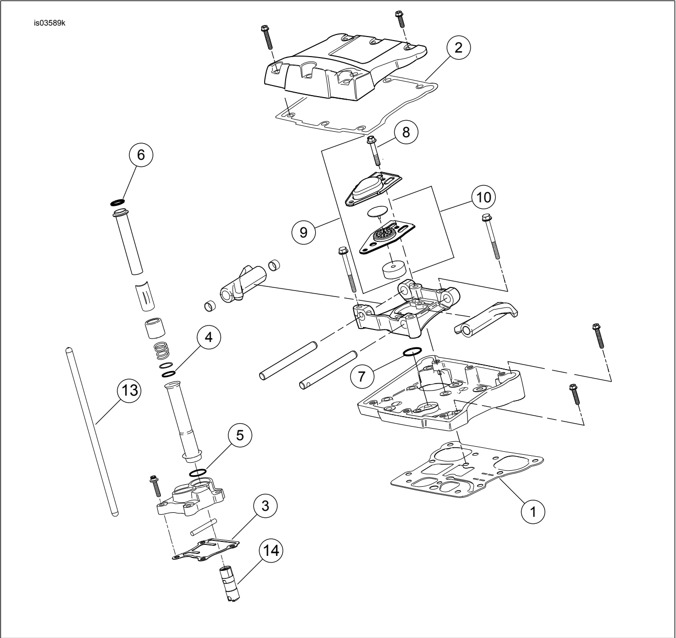
Şekil 2. Servis Parçaları: Screamin' Eagle TC 103 (1690 cc) Stage 4 Kiti
