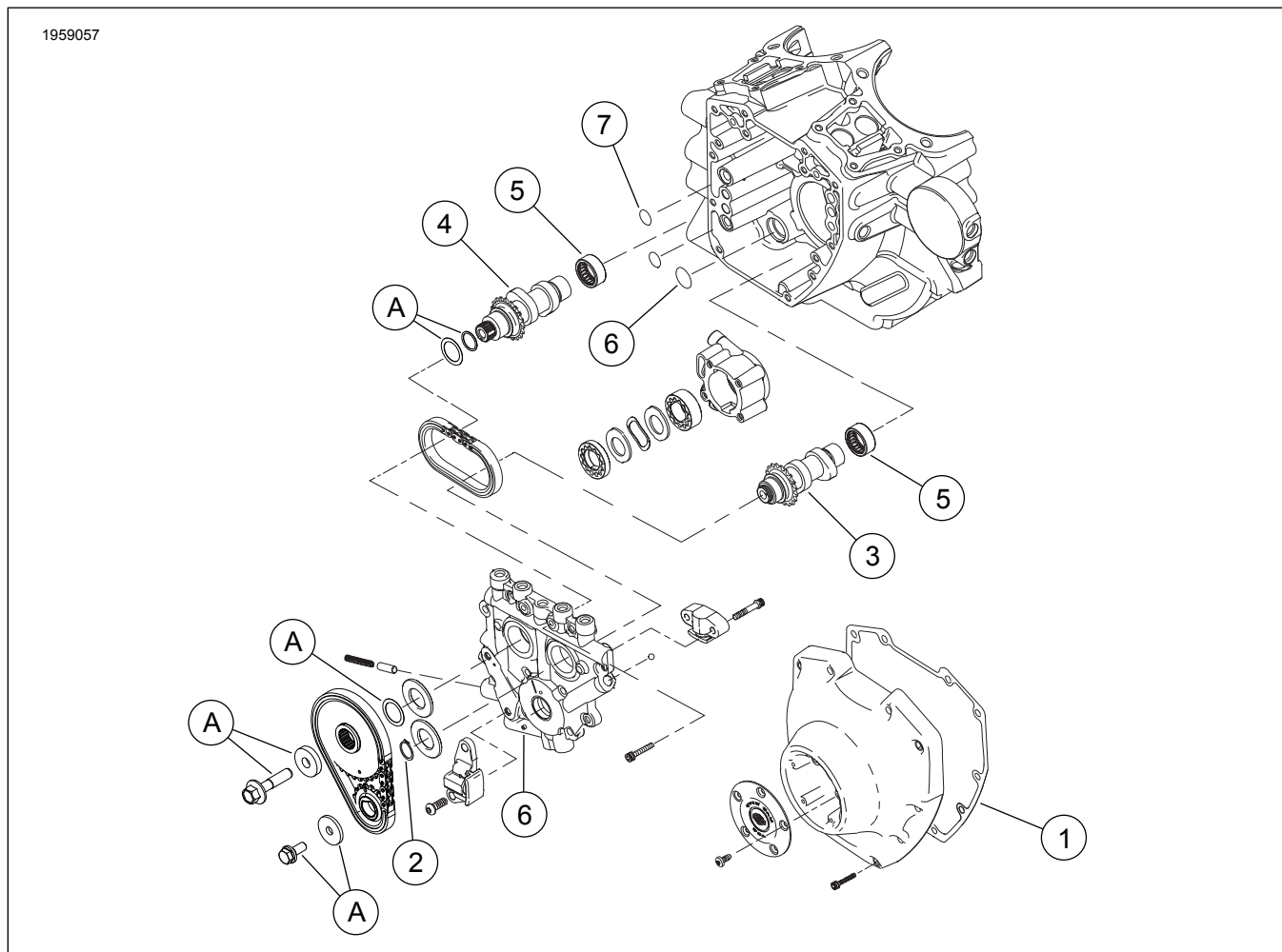
Slika 3. Servisni deli: Komplet Screamin' Eagle Pro 103 (1690 cc) Stage 4
