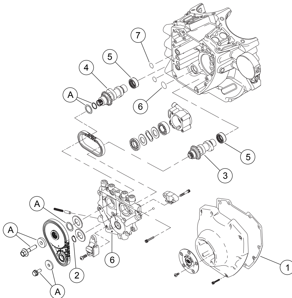
Εικόνα 3. Ανταλλακτικά: Κιτ Screamin' Eagle Pro 103 (1690 cc) Βαθμίδα 4
