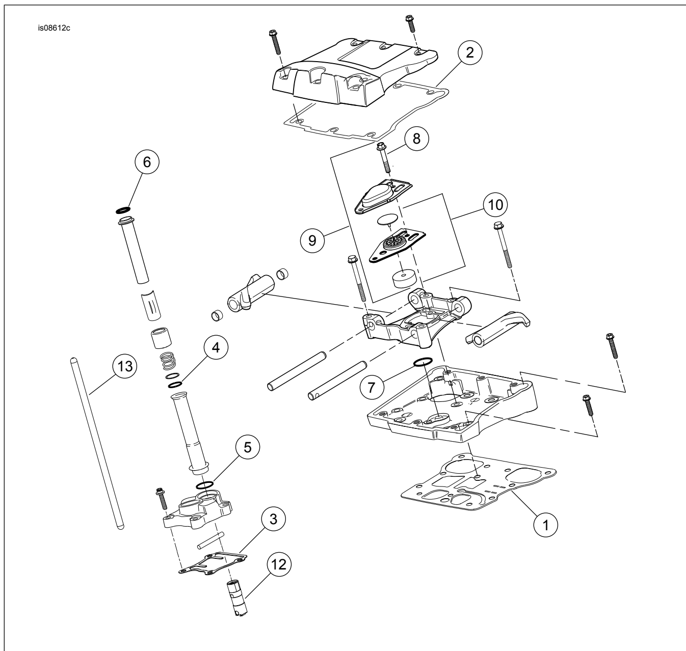
Фигура 2. Части за обслужване: Състезателен комплект Screamin' Eagle Twin Cam 110 (1800 cc) Stage V
