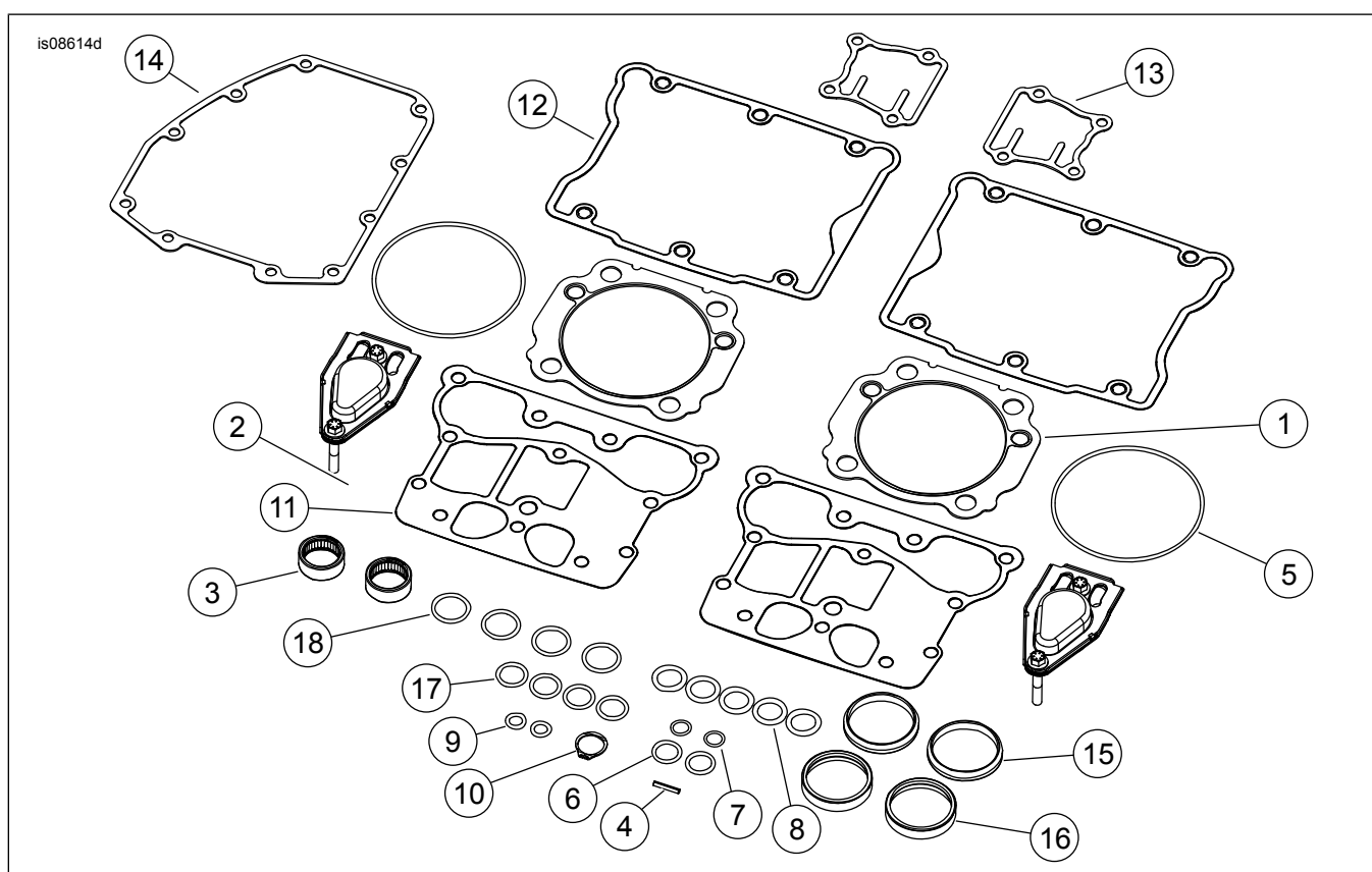
Фигура 4. Части за обслужване: Състезателен комплект Screamin' Eagle Twin Cam 110 (1800 cc) Stage V
