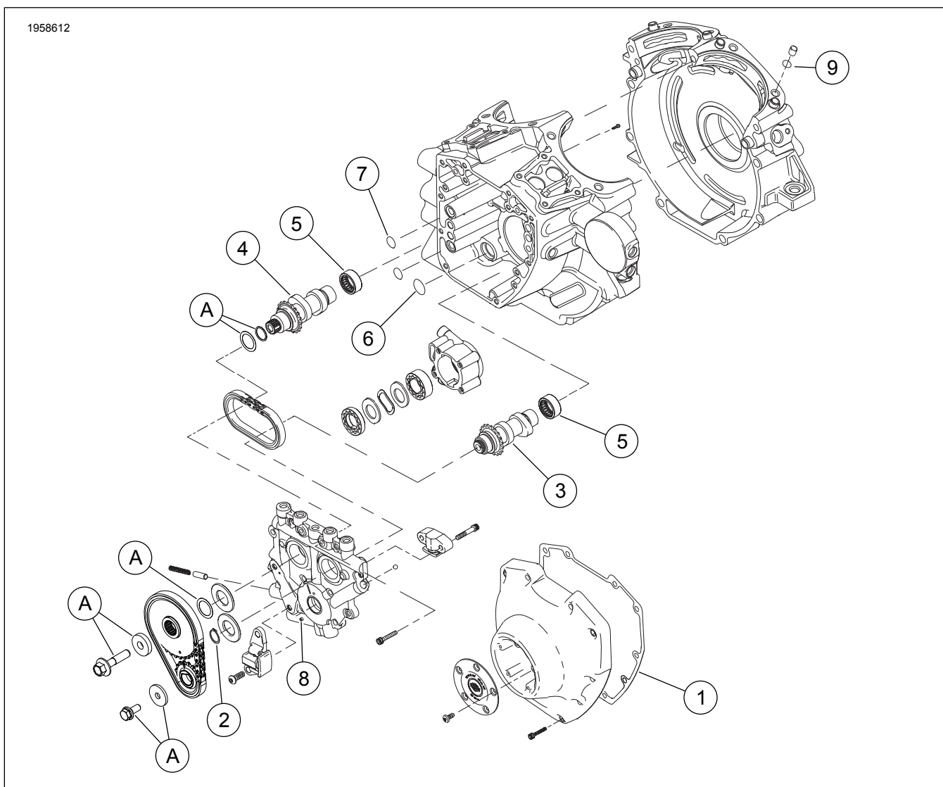
Фигура 3. Части за обслужване: Състезателен комплект Screamin' Eagle Twin Cam 110 (1800 cc) Stage V
