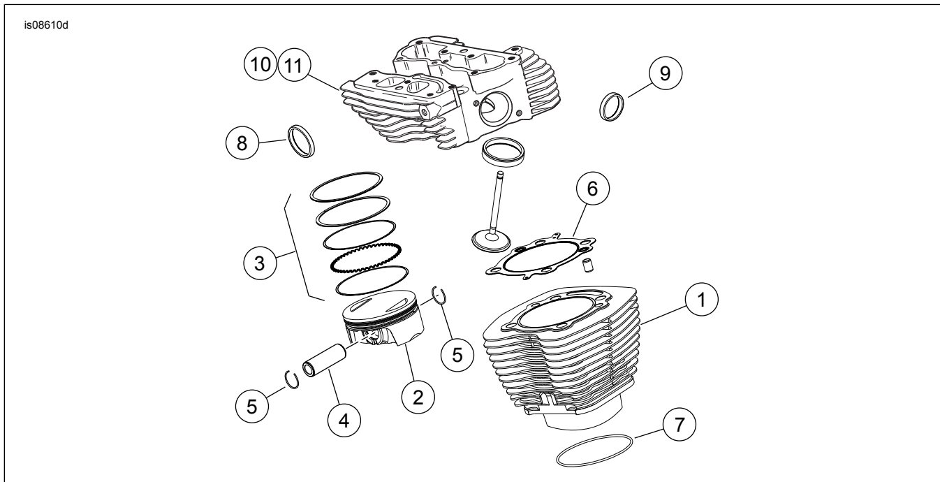
Фигура 1. Части за обслужване: Състезателен комплект Screamin' Eagle Twin Cam 110 (1800 cc) Stage V
