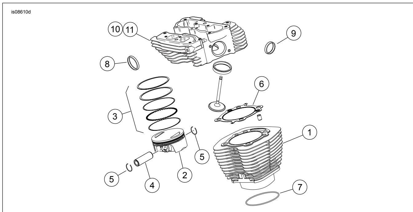
Joonis 1. Hooldatavad osad: Screamin' Eagle Twin Cam 110 (1800 cc) 5. etapi võistluskomplekt
