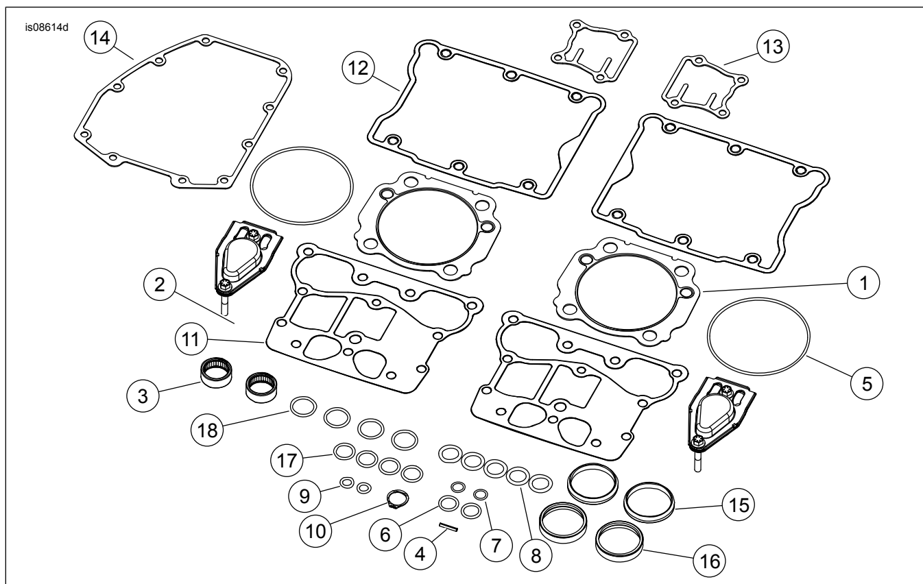
Joonis 4. Hooldatavad osad: Screamin' Eagle Twin Cam 110 (1800 cc) 5. etapi võistluskomplekt
