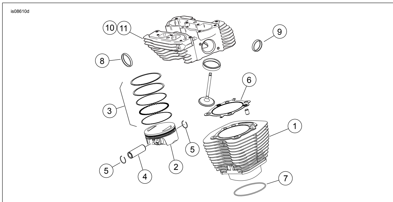
Attēls 1 Apkopes daļas: Screamin' Eagle Twin Cam 110 (1800 cc) V posma sacīkšu komplekts
