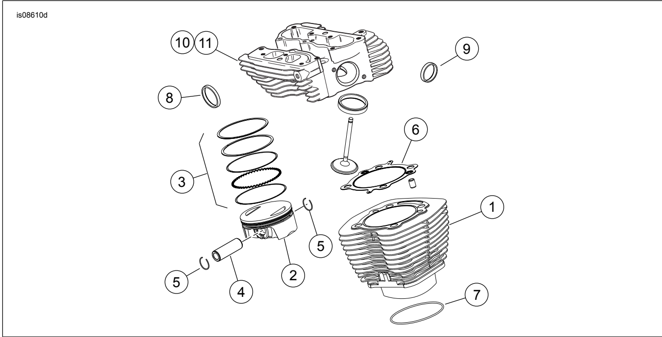
Şekil 1. Servis Parçaları: Screamin' Eagle Twin Cam 110 (1800 cc) Stage V Yarış Kiti
