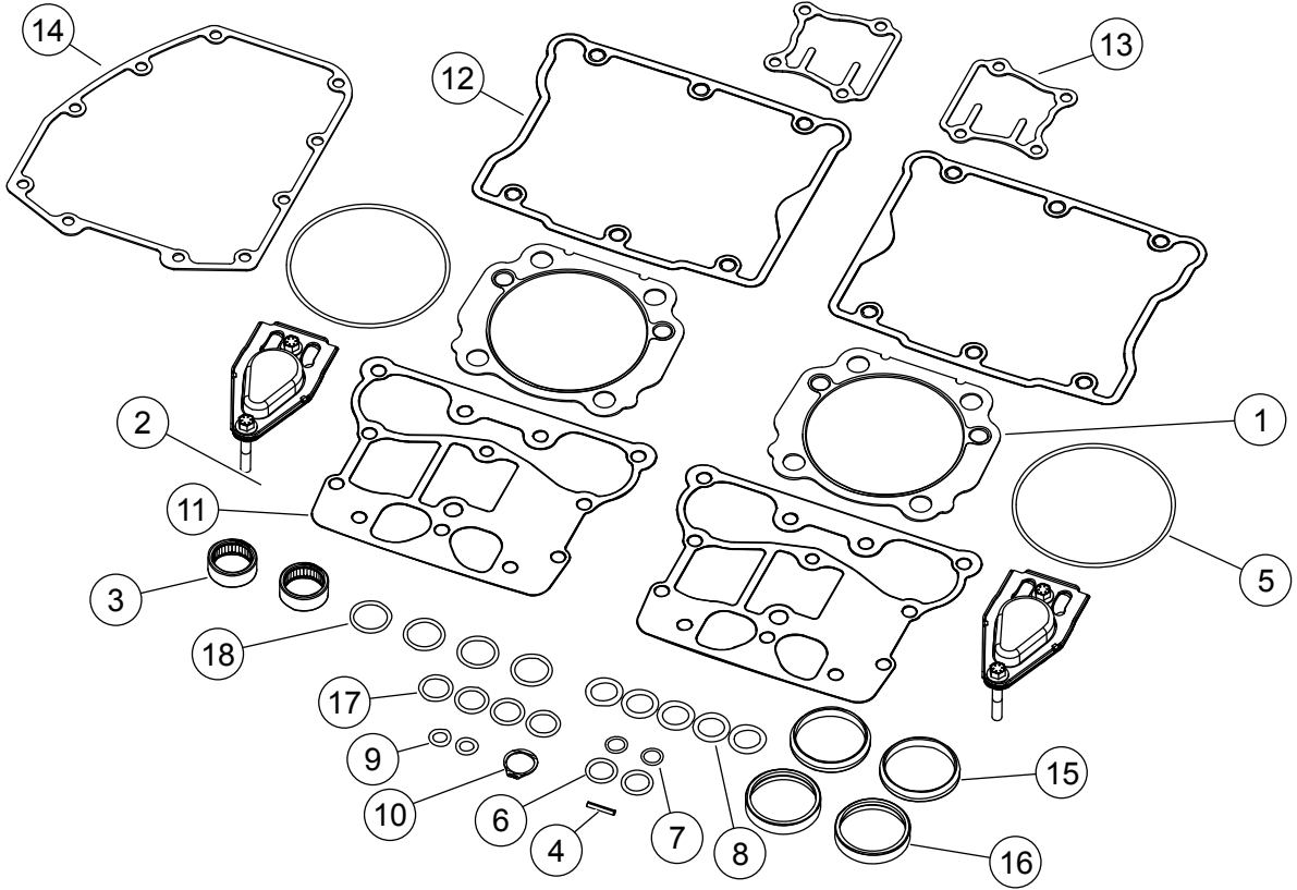
Şekil 4. Servis Parçaları: Screamin' Eagle Twin Cam 110 (1800 cc) Stage V Yaris Kiti
