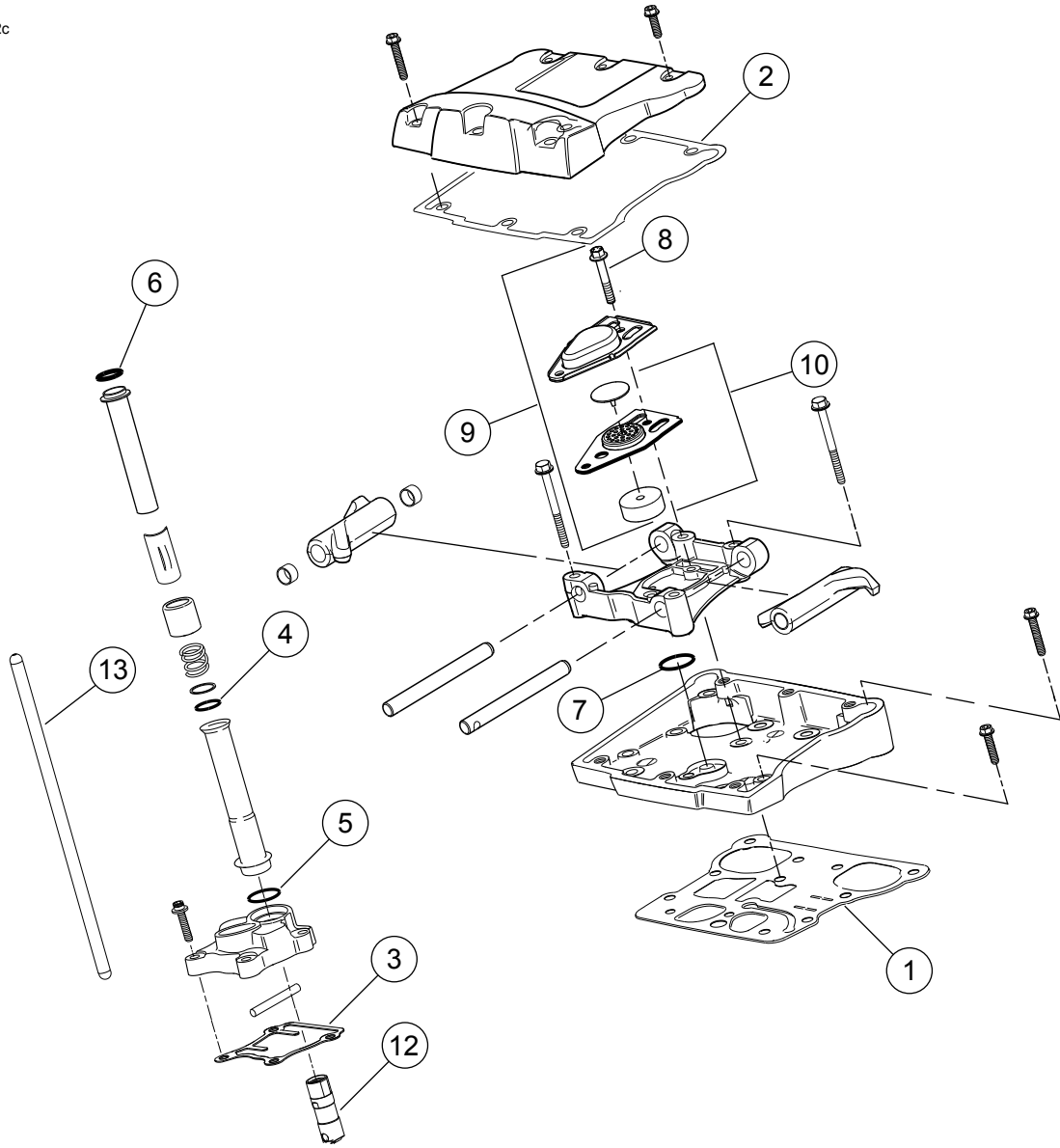
Şekil 2. Servis Parçaları: Screamin' Eagle Twin Cam 110 (1800 cc) Stage V Yariş Kiti
