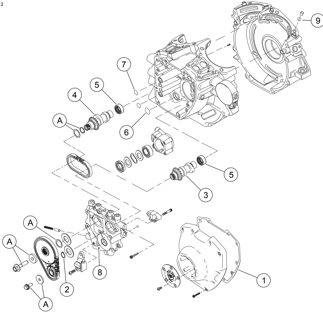
Şekil 3. Servis Parçaları: Screamin' Eagle Twin Cam 110 (1800 cc) Stage V Yariş Kiti
