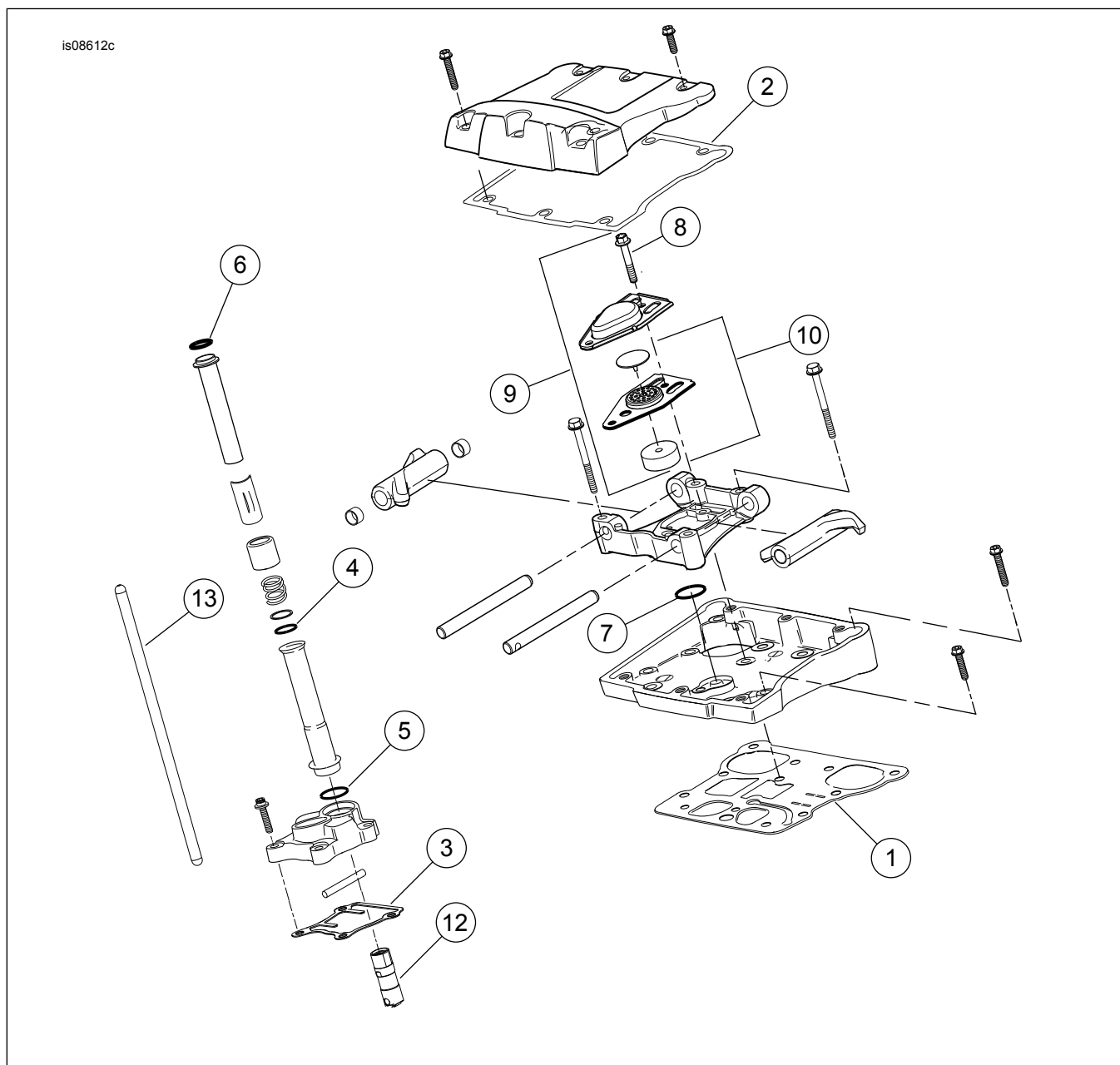
Ilustrace 2. Servisní díly: Závodní sada Screamin' Eagle Twin Cam 110 (1800 cm3) Stage V
