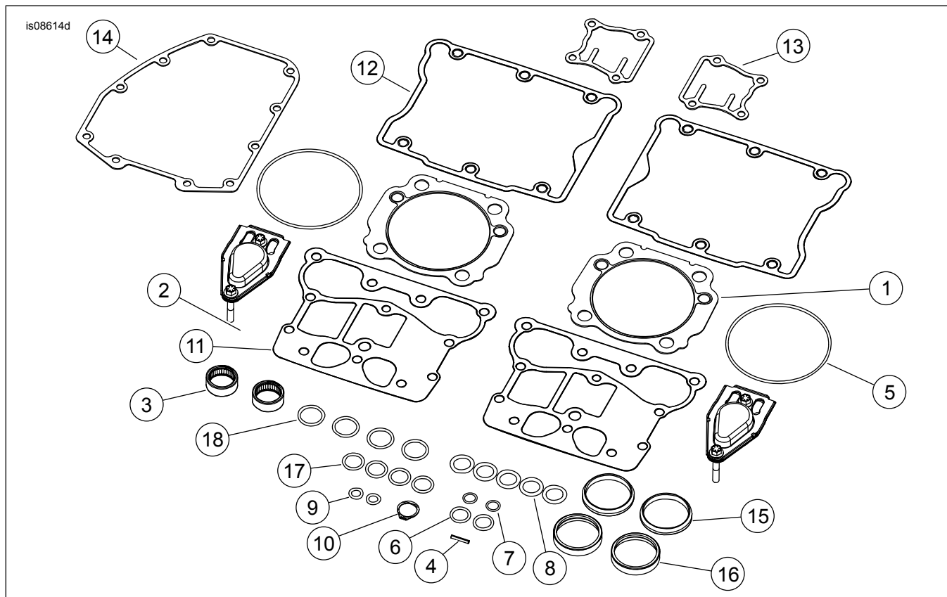
Ilustrace 4. Servisní díly: Závodní sada Screamin' Eagle Twin Cam 110 (1800 cm3) Stage V
