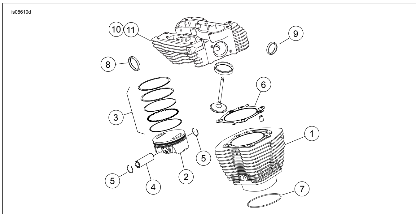
Ilustrace 1. Servisní díly: Závodní sada Screamin' Eagle Twin Cam 110 (1800 cm3) Stage V
