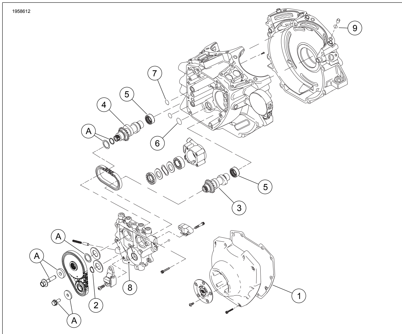
Ilustrace 3. Servisní díly: Závodní sada Screamin' Eagle Twin Cam 110 (1800 cm3) Stage V
